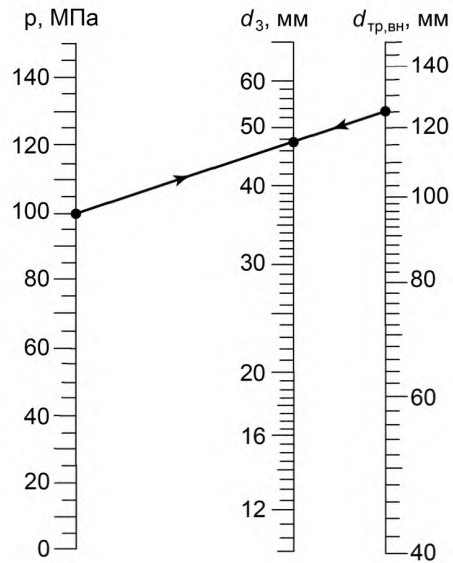
Рисунок 5 — Номограмма для определения диаметра заряда ФТ типа ТШТ для обрыва бурильных труб из алюминиевого сплава
