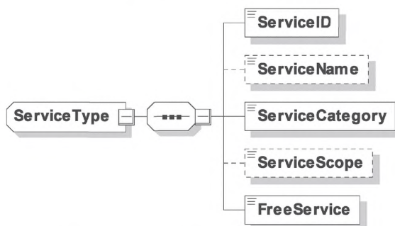
Рисунок 57 — Диаграмма — ServiceType
