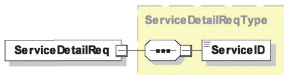
Рисунок 27 — Диаграмма — ServiceDetailReq
