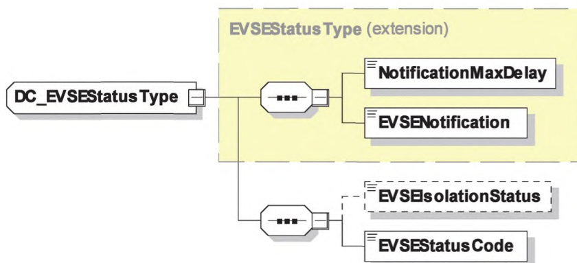
Рисунок 90 — Диаграмма — DC_EVSEStatusType
