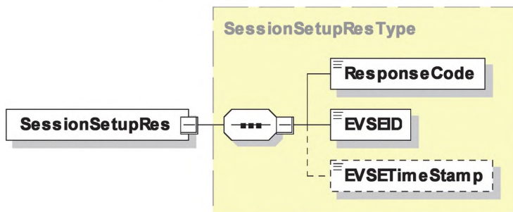
Рисунок 24 — Диаграмма — SessionSetupRes
