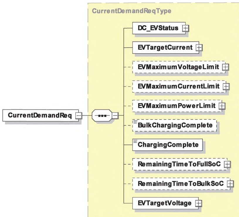
Рисунок 53 — Диаграмма — CurrentDemandReq
