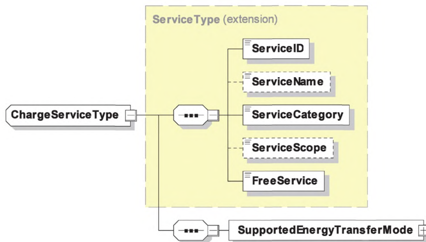
Рисунок 59 — Диаграмма — ChargeServiceType
