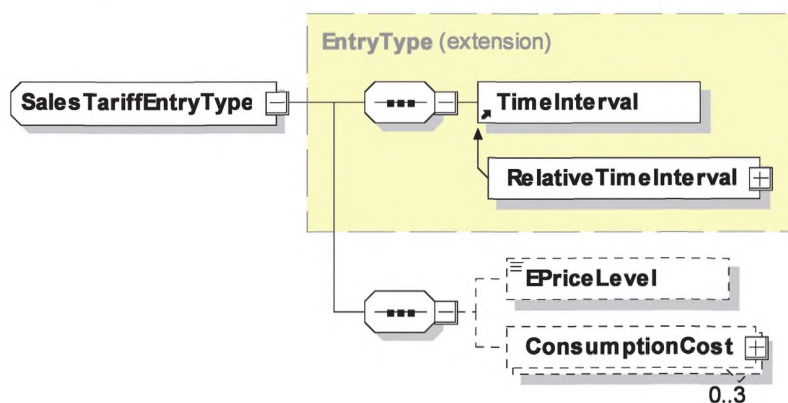
Рисунок 73 — Диаграмма — SalesTariffEntryType
