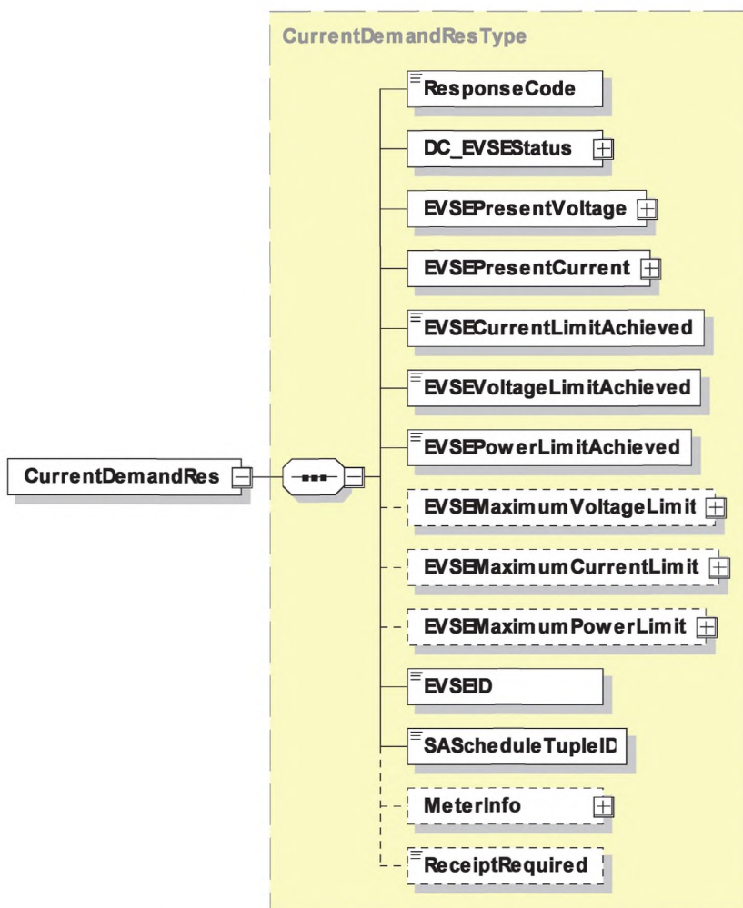
Рисунок 54 — Диаграмма — CurrentDemandRes
