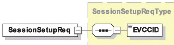
Рисунок 23 — Диаграмма — SessionSetupReq
