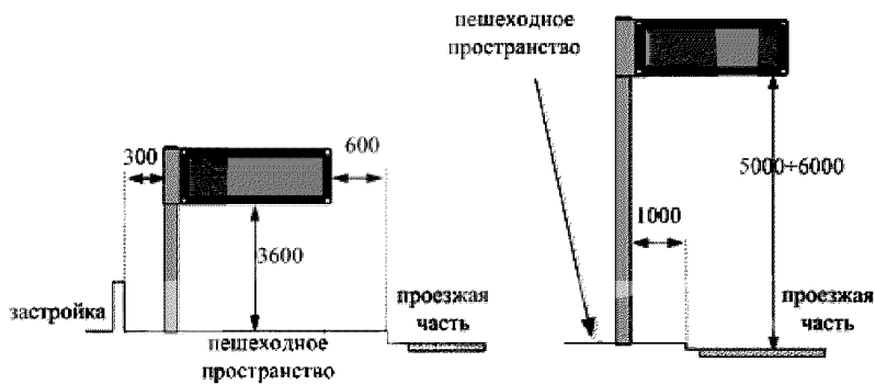
Рисунок 5.3 – Параметры размещения средств отображения динамической информации в населенных пунктах (размеры приведены в миллиметрах)
