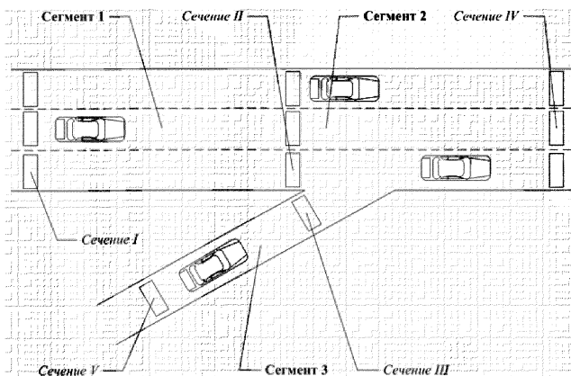
Рисунок 7.3 – Модель фрагмента УДС с примыканием к ОТП - четыре узла (2-х исходных – сечение I, сечение V; 1-го конечного - сечение IV; области слияния - сечения II-III; - три сегмента (сегмент I + сегмент 2 – основная магистраль; сегмент 3 – примыкание от ОТП).
