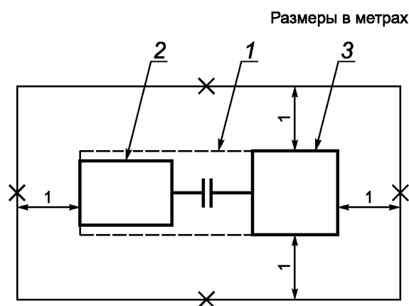
a) Медианная плоскость измерительной поверхности
