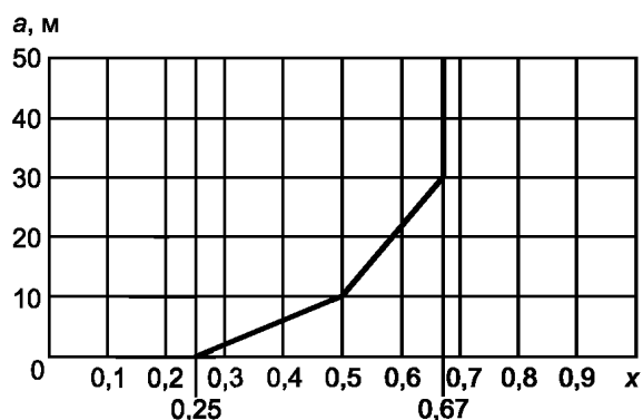
Рисунок А.2 — График для определения значения коэффициента x при зональном действии ветра
