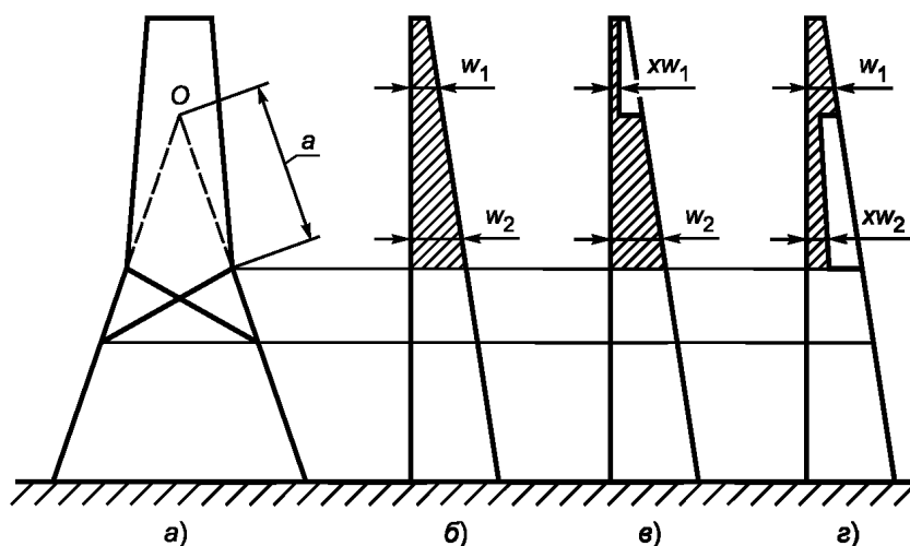
а) — условная схема башни с точкой схода поясов O ; б) — расчетная эпюра ветровой нагрузки на башню; в) — эпюра ветровой нагрузки на башню с учетом уменьшения ветровой нагрузки на участке выше схода поясов; г) — эпюра ветровой нагрузки на башню с учетом уменьшения ветровой нагрузки на участке ниже схода поясов
