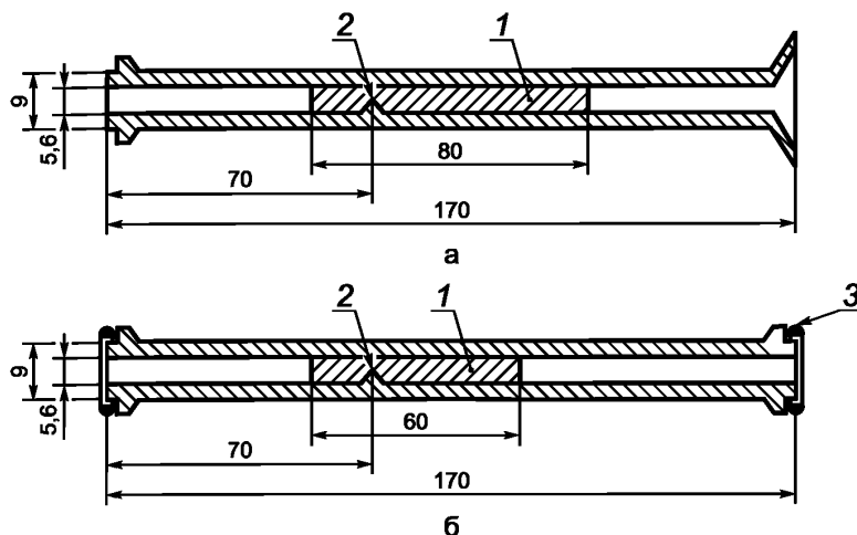
1 — нить из сплава золото/платина; 2 — выступ; 3 — уплотнительное кольцо
