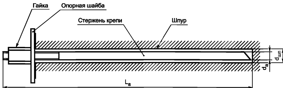
Рисунок 1 — Принципиальная схема крепи анкерной
