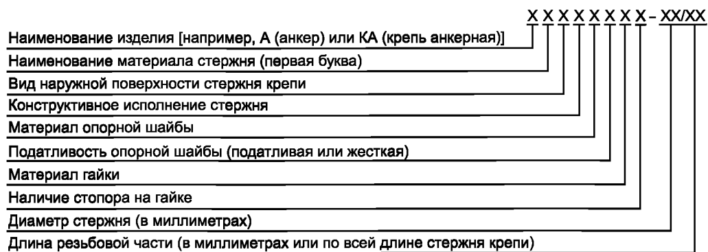
Рисунок 2 — Пример формирования обозначения крепи
