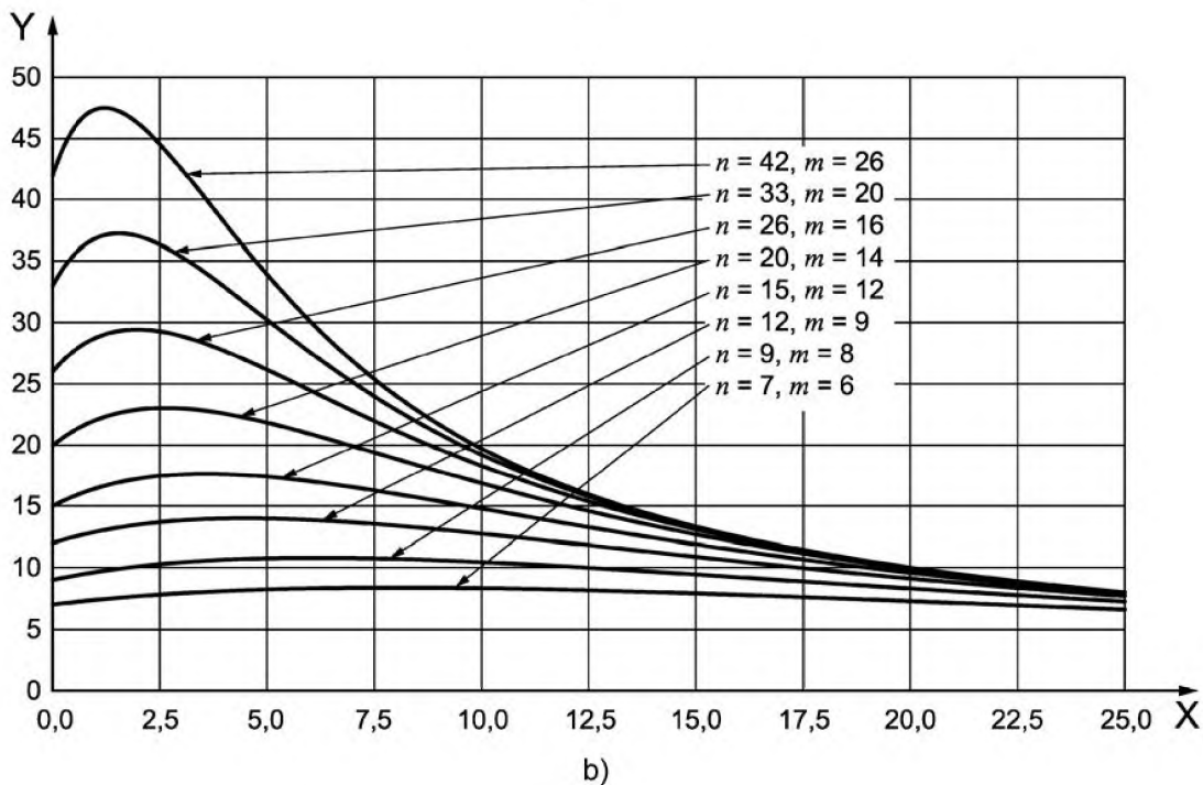
Рисунок 21 — Кривые среднего объема выборки для планов контроля доли несоответствующих единиц продукции, усеченный контроль с \alpha \leq 10\% и \beta \leq 10\%
