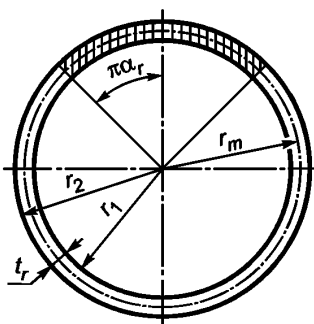
Рисунок 6 — Схема кольцевого сечения сталефибробетонного элемента, принимаемая при его расчете по прочности на изгиб
