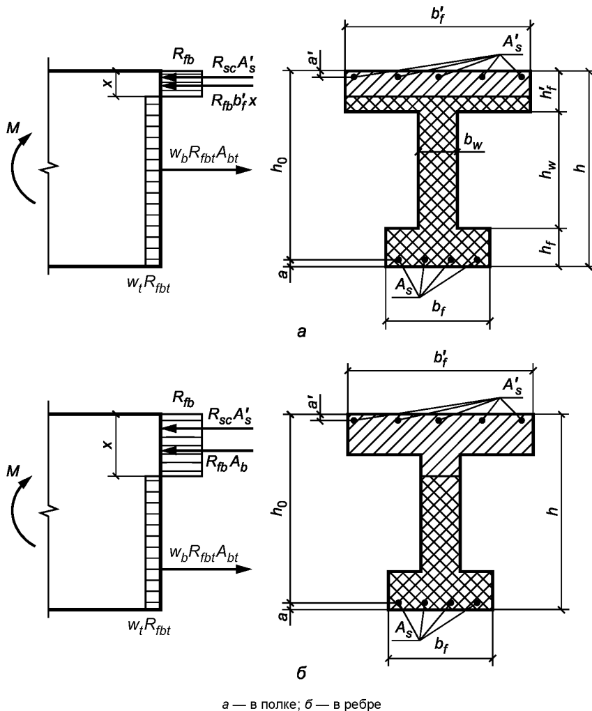
Рисунок 5 — Положение границы сжатой зоны в сечении изгибаемого сталефибробетонного элемента с арматурой
