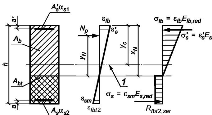
1 — уровень центра тяжести приведенного без учета растянутой зоны сталефибробетона поперечного сечения
