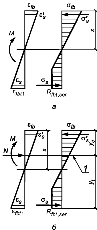
Рисунок 19 — Схема напряженно-деформированного состояния сечения элемента при проверке образования трещин при действии изгибающего момента (а) и изгибающего момента и продольной силы (б)
