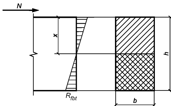
Рисунок 8 — Схема усилий и эпюра напряжений в сечении, нормальном к продольной оси внецентренно сжатого сталефибробетонного элемента, рассчитываемого по прочности с учетом сопротивления сталефибробетона растянутой зоны
