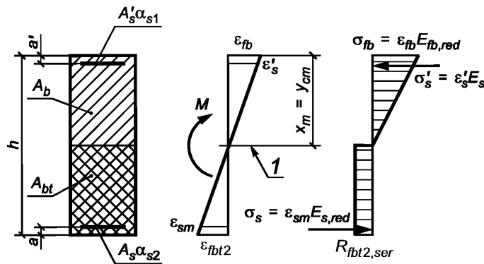
1 — уровень центра тяжести поперечного сечения
