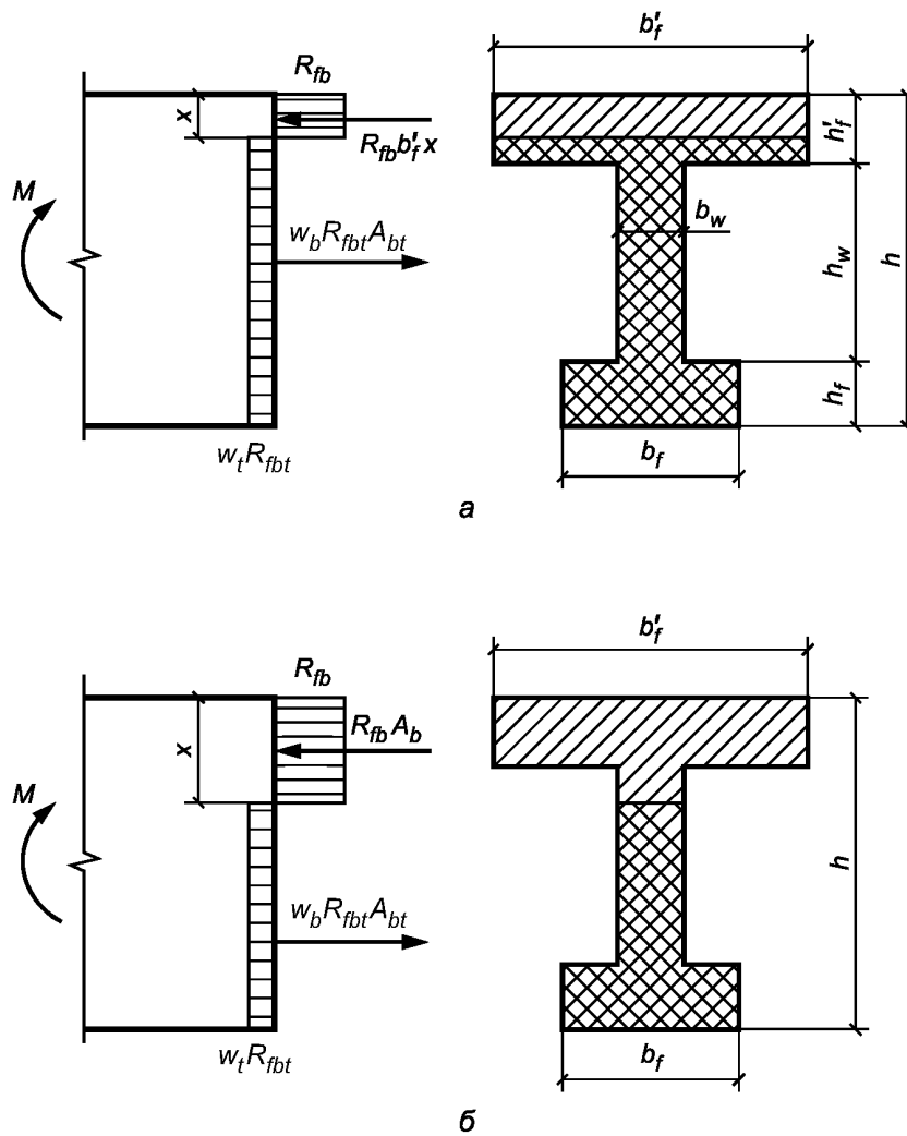
а — в полке; б — в ребре
