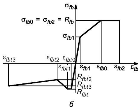
Рисунок 1 — Диаграммы деформирования сталефибробетона при сжатии и растяжении
