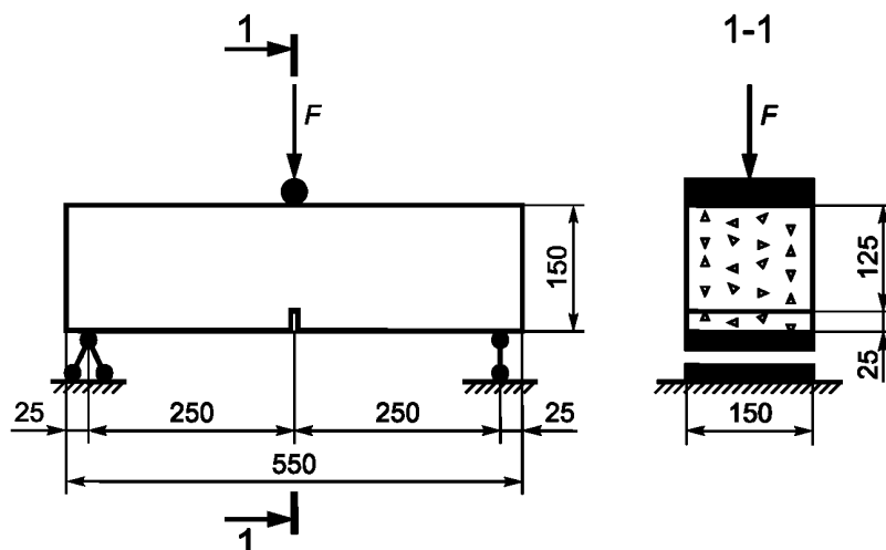
Рисунок Б.1 — Схема испытания образца
