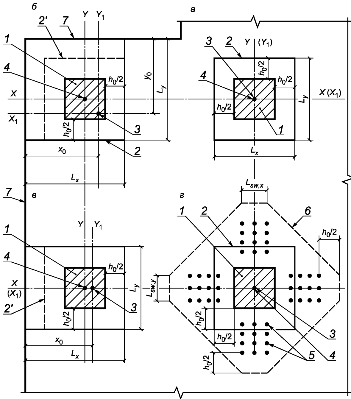
а — площадка приложения нагрузки внутри плоского элемента; б, в — то же, у края плоского элемента; г — при крестообразном расположении поперечной арматуры; 1 — площадь приложения нагрузки; 2 — расчетный контур поперечного сечения; 2' — второй вариант расположения расчетного контура; 3 — центр тяжести расчетного контура (место пересечения осей X_1 и Y_1 ); 4 — центр тяжести площадки приложения нагрузки (место пересечения осей X и Y ); 5 — поперечная арматура; 6 — контур расчетного поперечного сечения без учета в расчете поперечной арматуры; 7 — граница (край) плоского элемента
