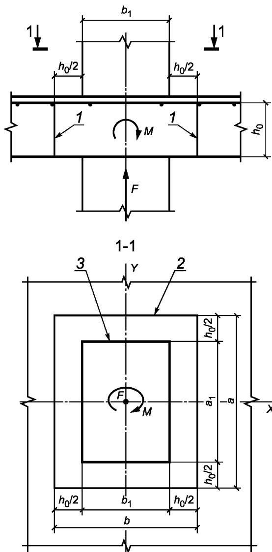
Рисунок 17 — Схема для расчета сталефибробетонных элементов без поперечной арматуры на продавливание
