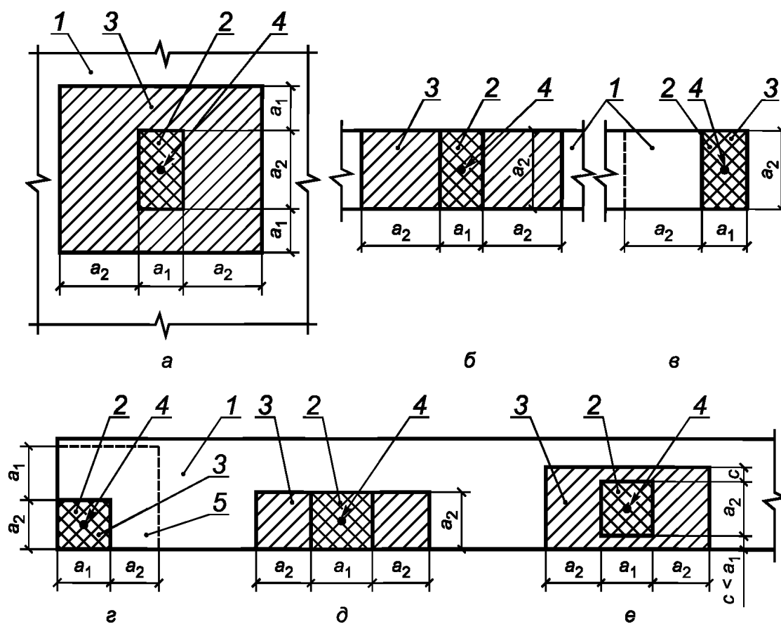
а — вдали от краев элемента; б — по всей ширине элемента; в — у края (торца) элемента по всей его ширине; г — на углу элемента; д — у одного края элемента; е — вблизи одного края элемента; 1 — элемент, на который действует местная нагрузка; 2 — площадь смятия A_{fb,loc} ; 3 — максимальная расчетная площадь A_{fb,max} ; 4 — центр тяжести площадей A_{fb,loc} и A_{fb,max} ; 5 — минимальная зона армирования сетками, при которой косвенное армирование учитывается в расчете
