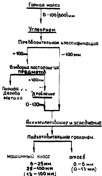
Рис.1. типовая схема операций углеподготовки перед обогащением.
