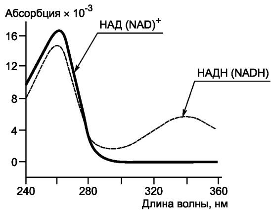
Рисунок А.1 — Различие в спектрах поглощения между окисленной и восстановленной формами никотинамиддениндинуклеотида (НАДН) в ультрафиолетовой области спектра
