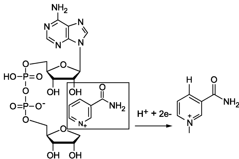
Рисунок А.2 — Реакция обратимого окисления никотинамиддениндинуклеотида
