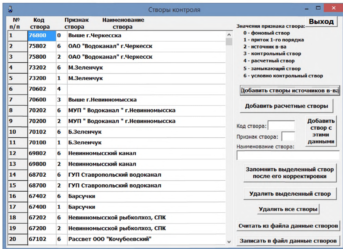
Рисунок Г.8 – Пример экранной формы программы с назначенными признаками створов на р. Кубань
