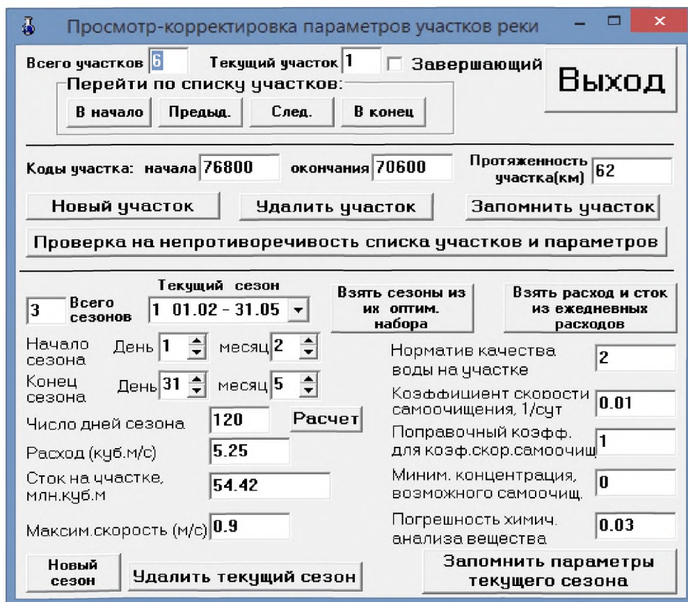
Рисунок Б.4 – Пример заполненной данными экранной формы программы по отдельному выделенному участку реки
