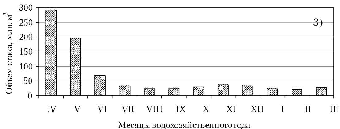
Рис. А.26. Расчетное внутригодовое распределение стока реки Луга — ст. Толмачево для года обеспеченностью P=90\% ; 1 — метод среднего распределения стока за годы характерной градации водности, 2 — метод реального года, 3 — метод компоновки
