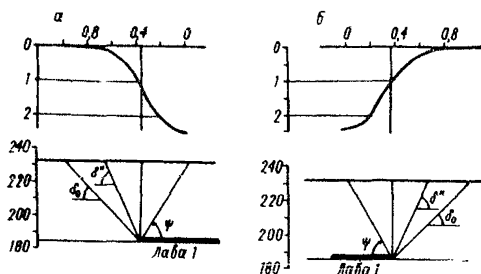
Рис. 21. Вспомогательные разрезы и графики оседаний для профиля по линии U_1-U_1 (над лавой I)
