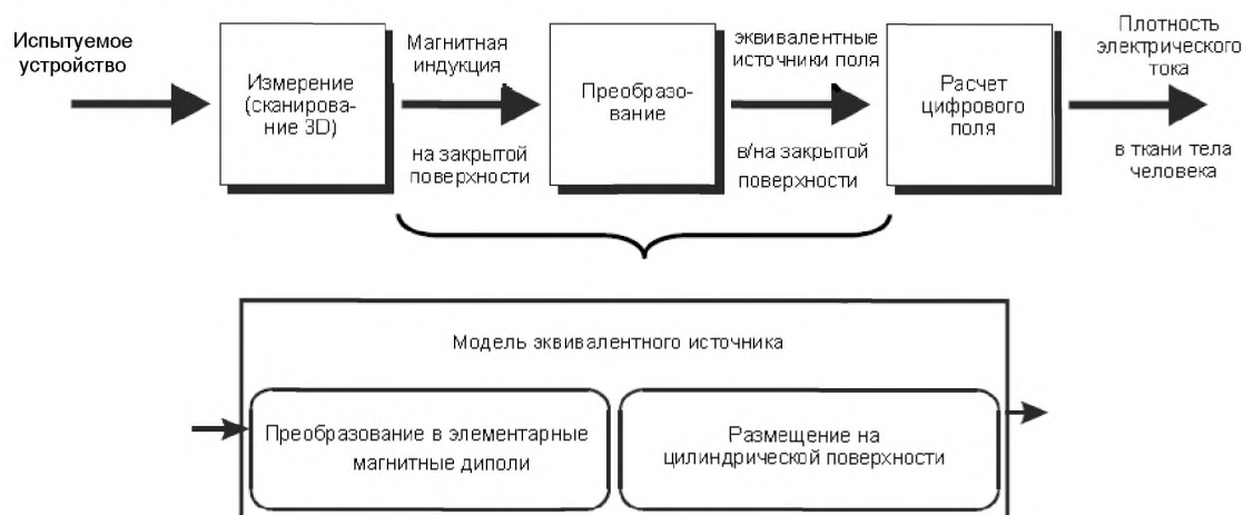
Рисунок С.6 – Блок-схема метода
