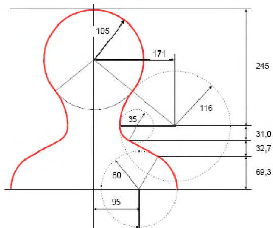
Рисунок С.3б – Детальный чертеж модели головы и плеч
