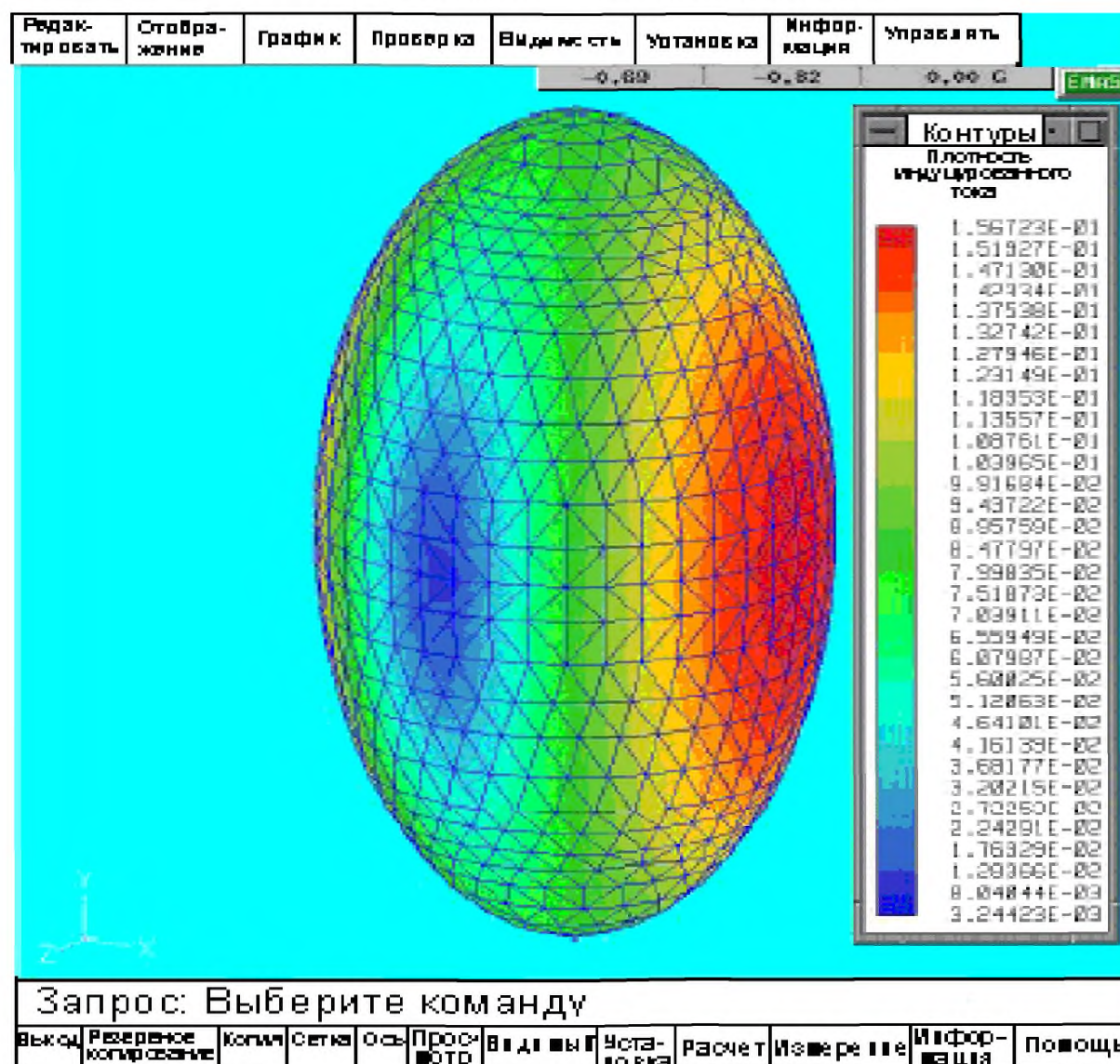
Рисунок С.12б – Плотность индуцированного тока
