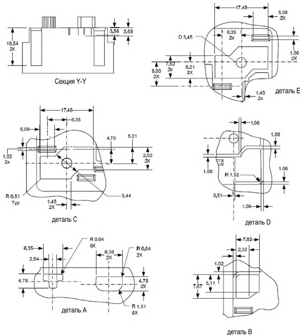
Рисунок 62 – Схема плоского разъема магистральной линии – геометрия
