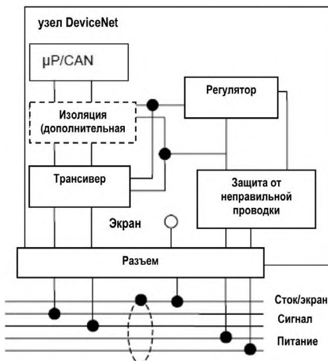
Рисунок 47 – Блок-схема физического слоя
