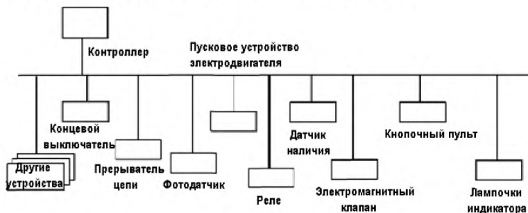
Рисунок 1 – Типовые интерфейсы DeviceNet между контроллерами и устройствами
