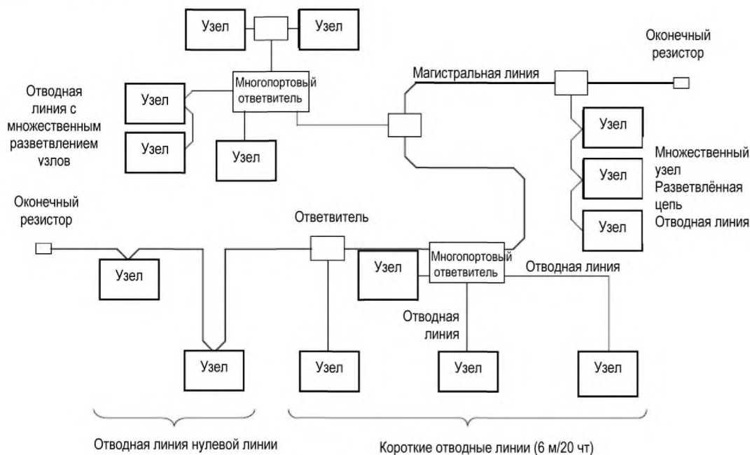
Рисунок 50 – Топология среды DeciceNet
