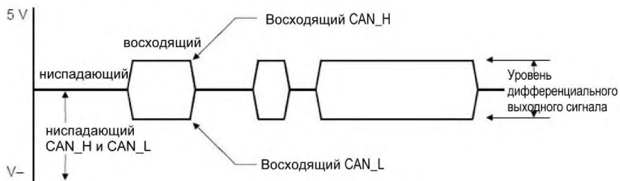
Рисунок 69 – Уровни передачи
