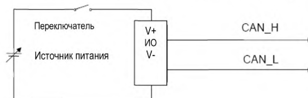
Рисунок 65 – Испытательная цепь включения питания
