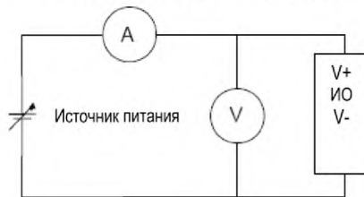
Рисунок 64 – Испытательная цепь потребления тока
