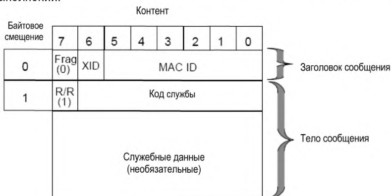
Рисунок 14 – Формат нефрагментированного сообщения-отклика об успешном выполнении
