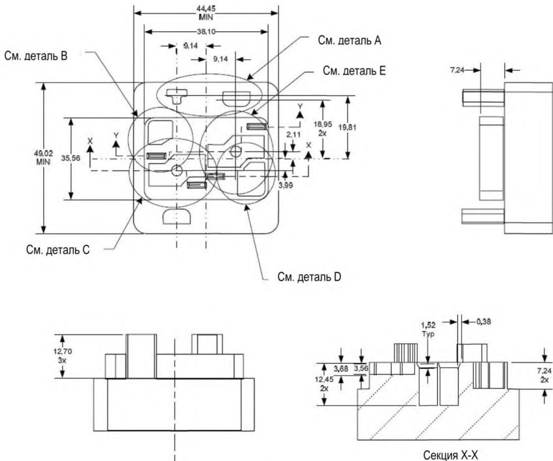
Рисунок 61 – Схема плоского разъема магистральной линии – разводка контактов
