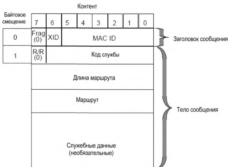
Рисунок 13 – Формат явного нефрагментированного сообщения-запроса, значение 4
