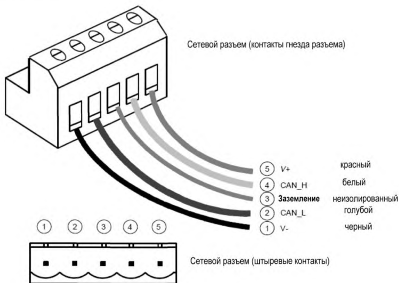
Рисунок 57 – Разводка контактов сетевого разъема
