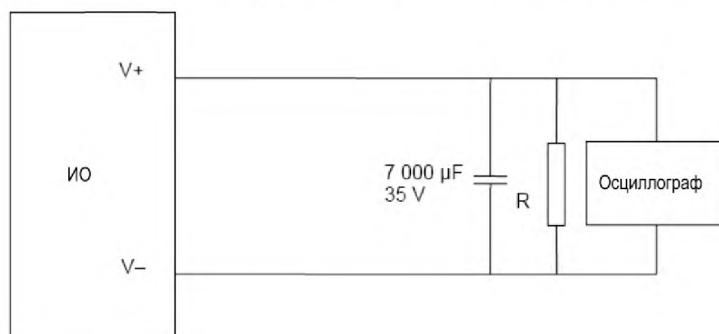
Рисунок 63 – Испытательная цепь нарастания напряжения питания по времени
