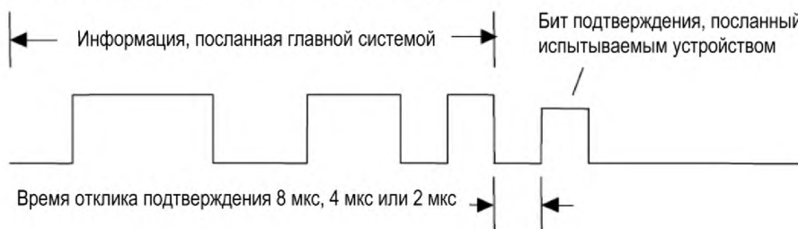
Рисунок 71 – Временная выдержка
