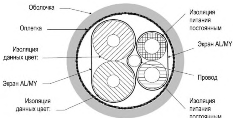
Рисунок 53 – Тонкий кабель: физическая конфигурация
