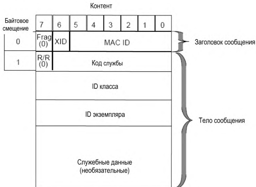
Рисунок 12 – Формат явного нефрагментированного сообщения-запроса, значения 0 – 3
