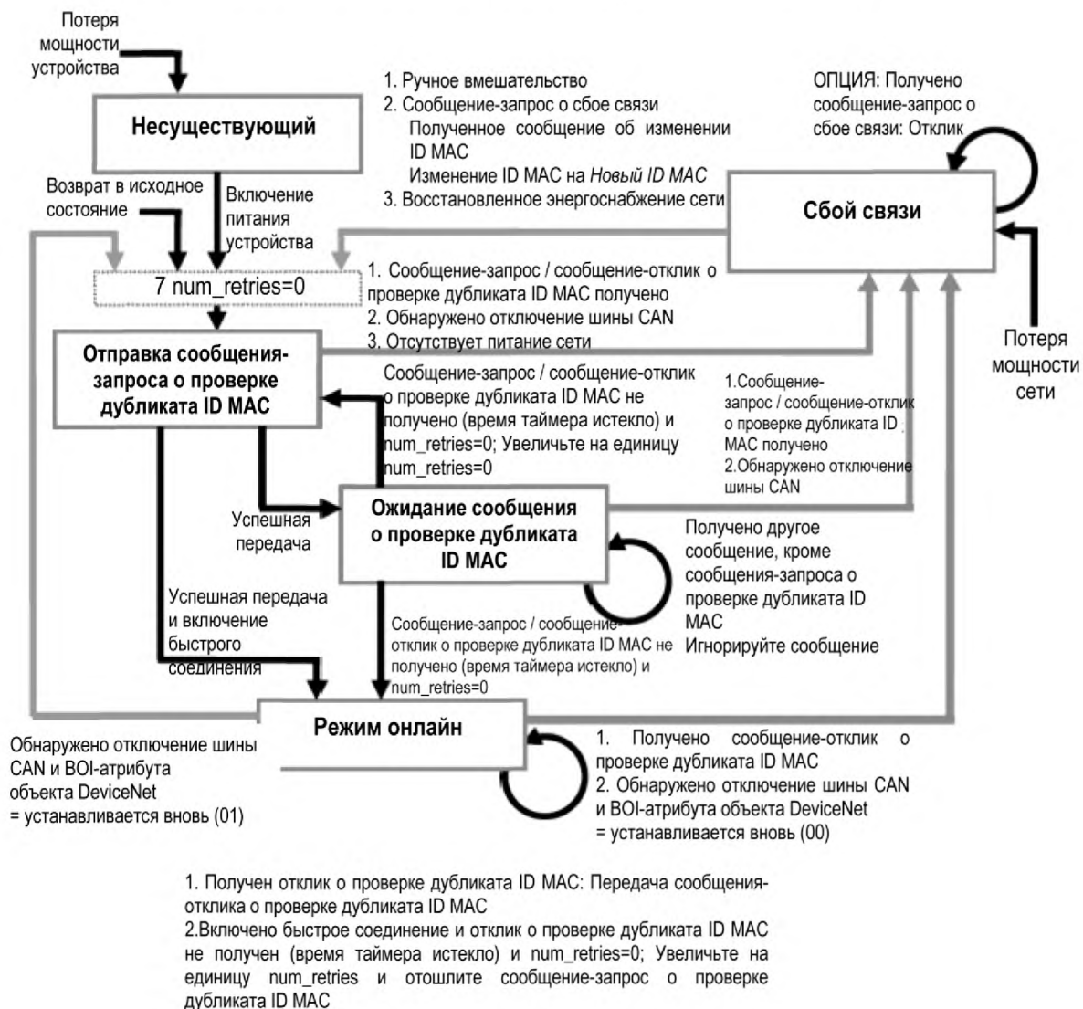
Рисунок 37 – Схема передачи состояния доступа к каналу связи
