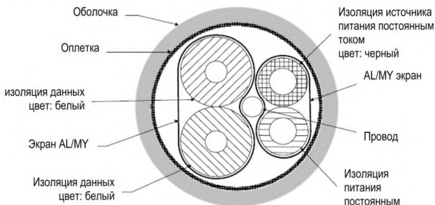
Рисунок 51 – Толстый кабель: физическая конфигурация
