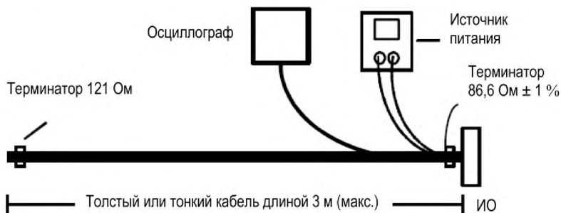
Рисунок 68 – Схема испытания уровня передачи
