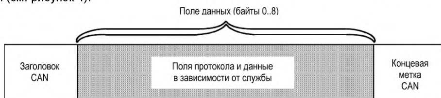
Рисунок 4 – Использование поля данных явного сообщения CAN
