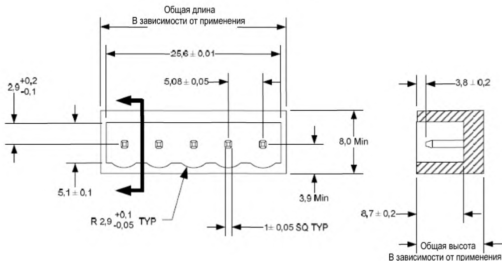
Рисунок 58 – Геометрия открытого разъема
