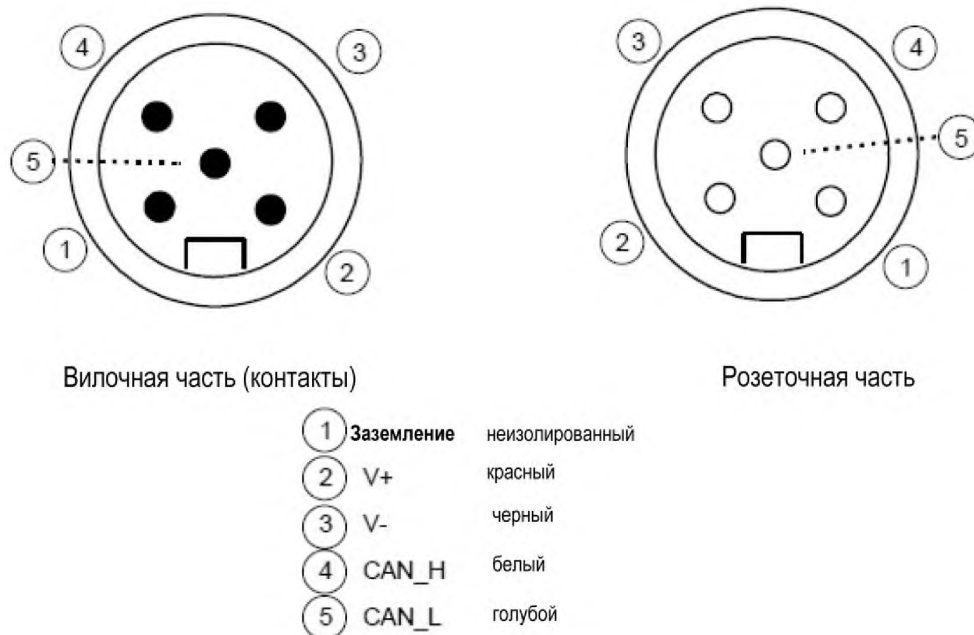
Рисунок 60 – Разводка контактов микро-разъема
