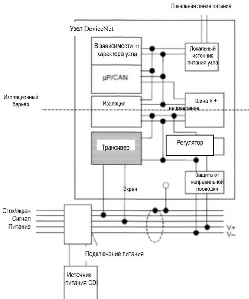
Рисунок 49 – Устройство, содержащее изолированный физический уровень
