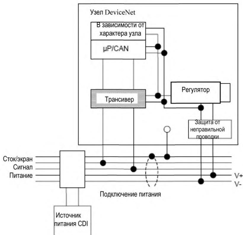
Рисунок 48 – Устройство, содержащее неизолированный физический уровень
