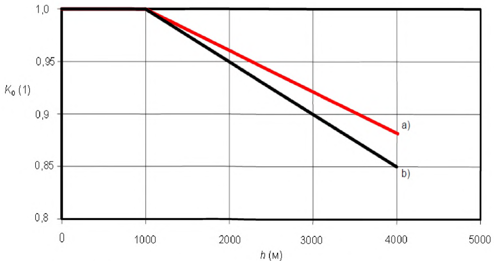
Рисунок 1 — Коэффициент коррективы высоты для превышения температуры
