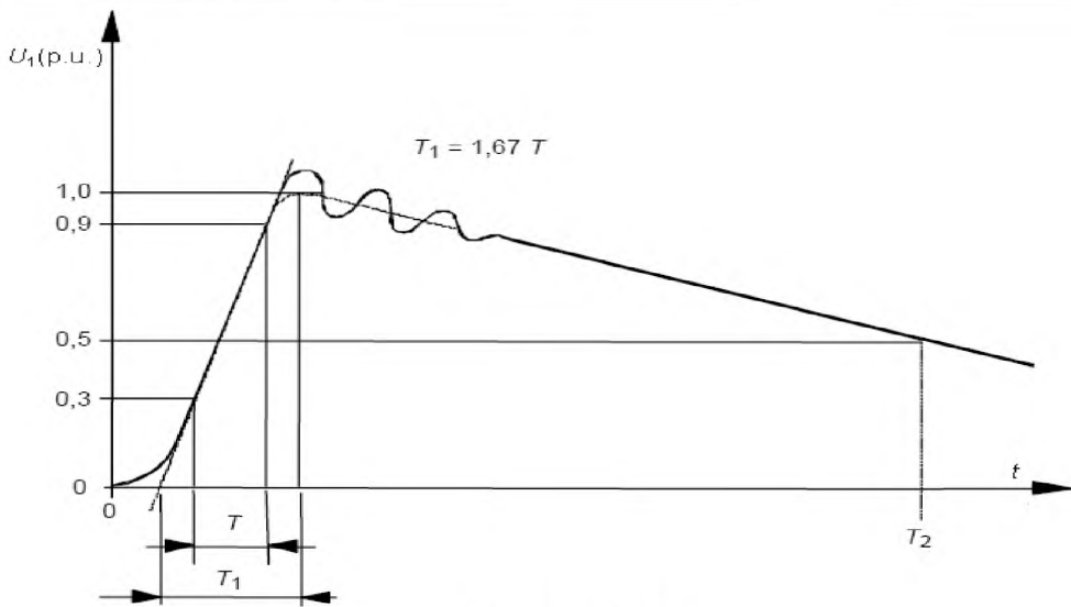
Форма импульса А
