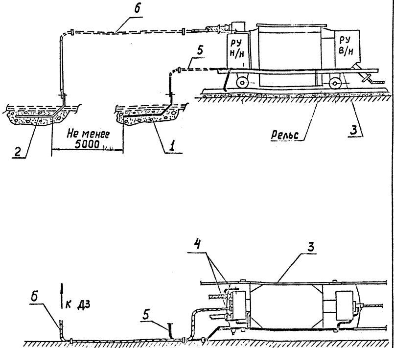
Рис. 7. Схема заземления передвижной подстанции и реле УАКИ.
