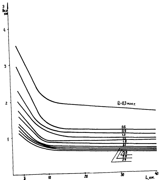
Усредненные показатели энергоемкости установок ТКИТ при \alpha = 0,5^\circ и \rho = 900 \text{ кг/м}^3
