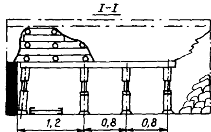
Рис. 17. Схема крепления с вы- кладкой деревянных клеток
