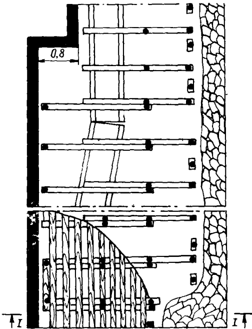
Рис. 16. Схема крепления с затяжкой кровли деревом
