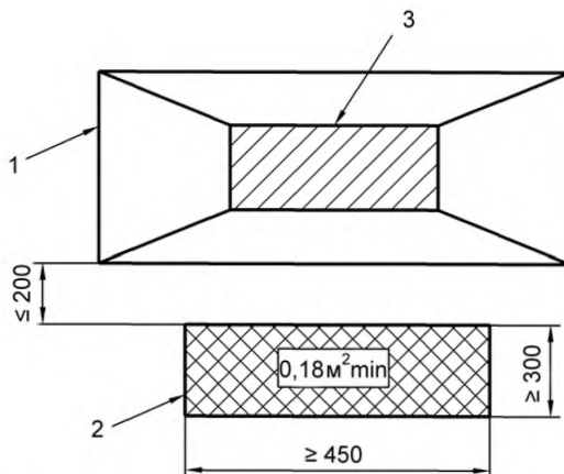
1 – бункер; 2 – платформа; 3 – зона дозирующего устройства
