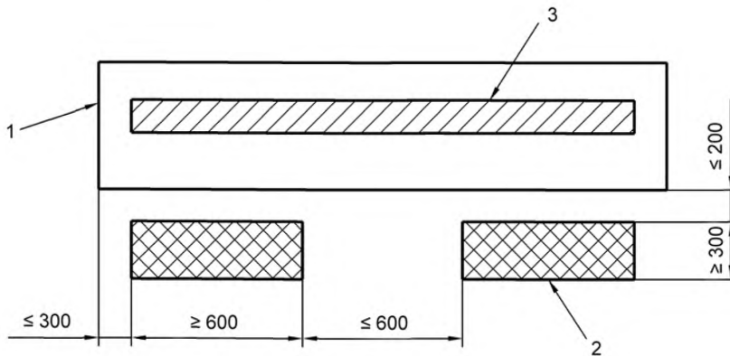
1 – бункер; 2 – платформа; 3 – зона дозирующего устройства
