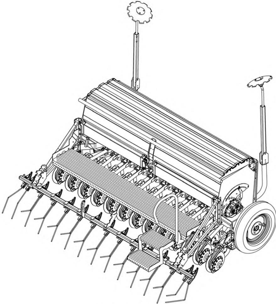
Рисунок А.1 – Механическая рядовая сеялка
