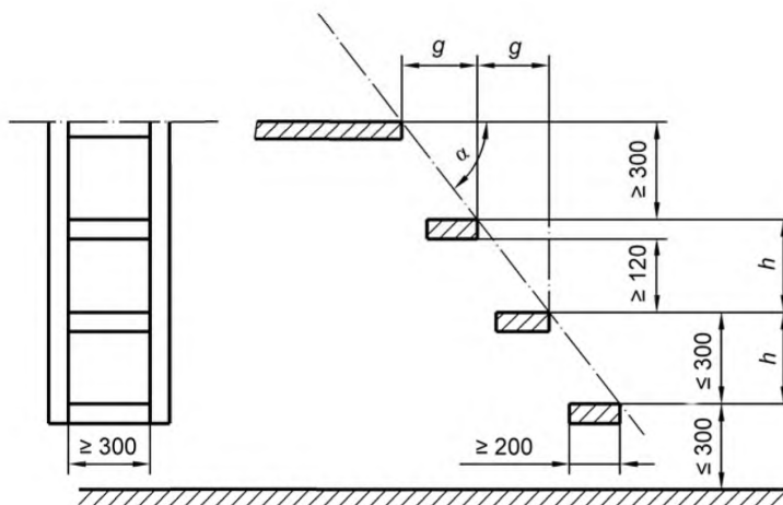
Рисунок 5 – Размеры средств доступа к месту ручной загрузки
