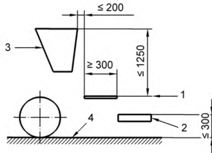
1 – платформа; 2 – ступенька; 3 – бункер, 4 – грунт
