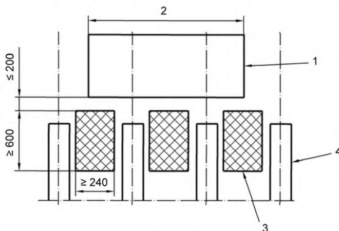
1 – контур проема бункера; 2 – ширина бункера; 3 – платформа; 4 – высеваящий аппарат Примечание – Минимальное число платформ зависит от ширины бункера (см. 5.5.1).
