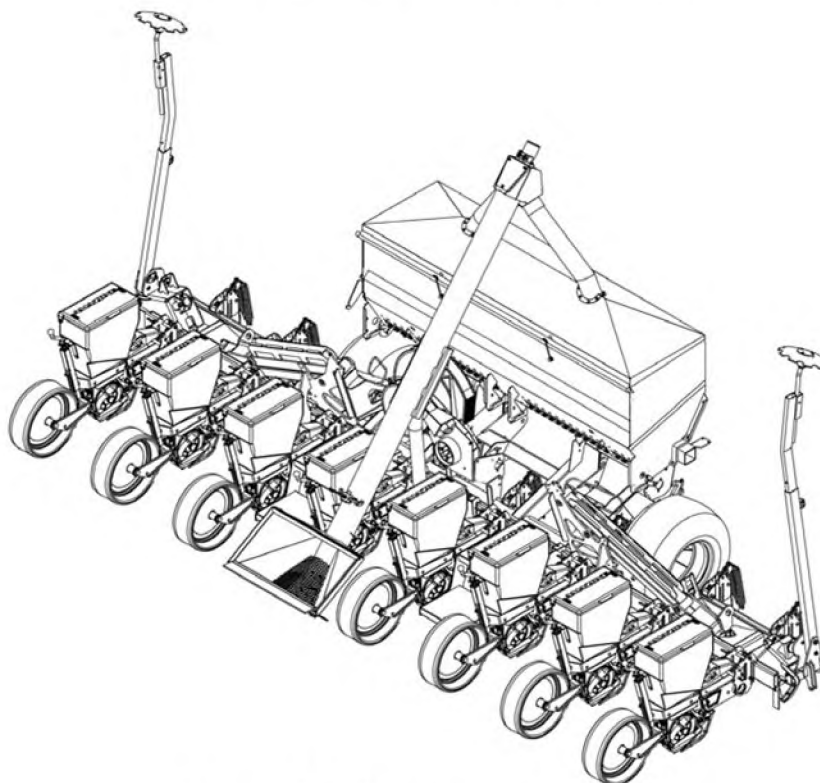
Рисунок А.3 – Сеялка точного высева
