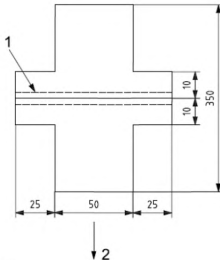
Рисунок В.1 — Образец для испытаний для измерения прочности на разрыв нижнего шва
