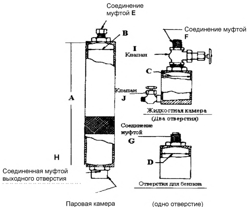
Размеры аппарата для давления паров
