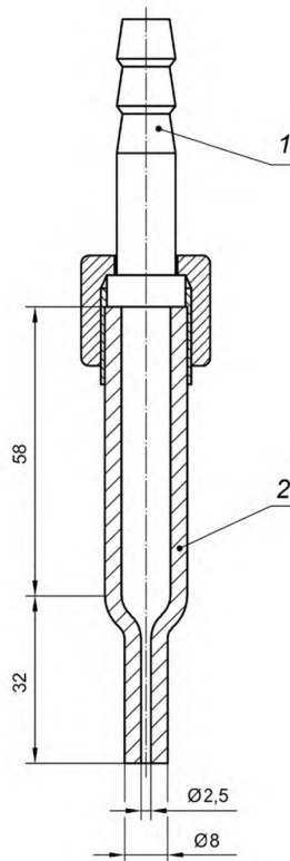
1 — соединительная трубка; 2 — пробоотборная трубка
