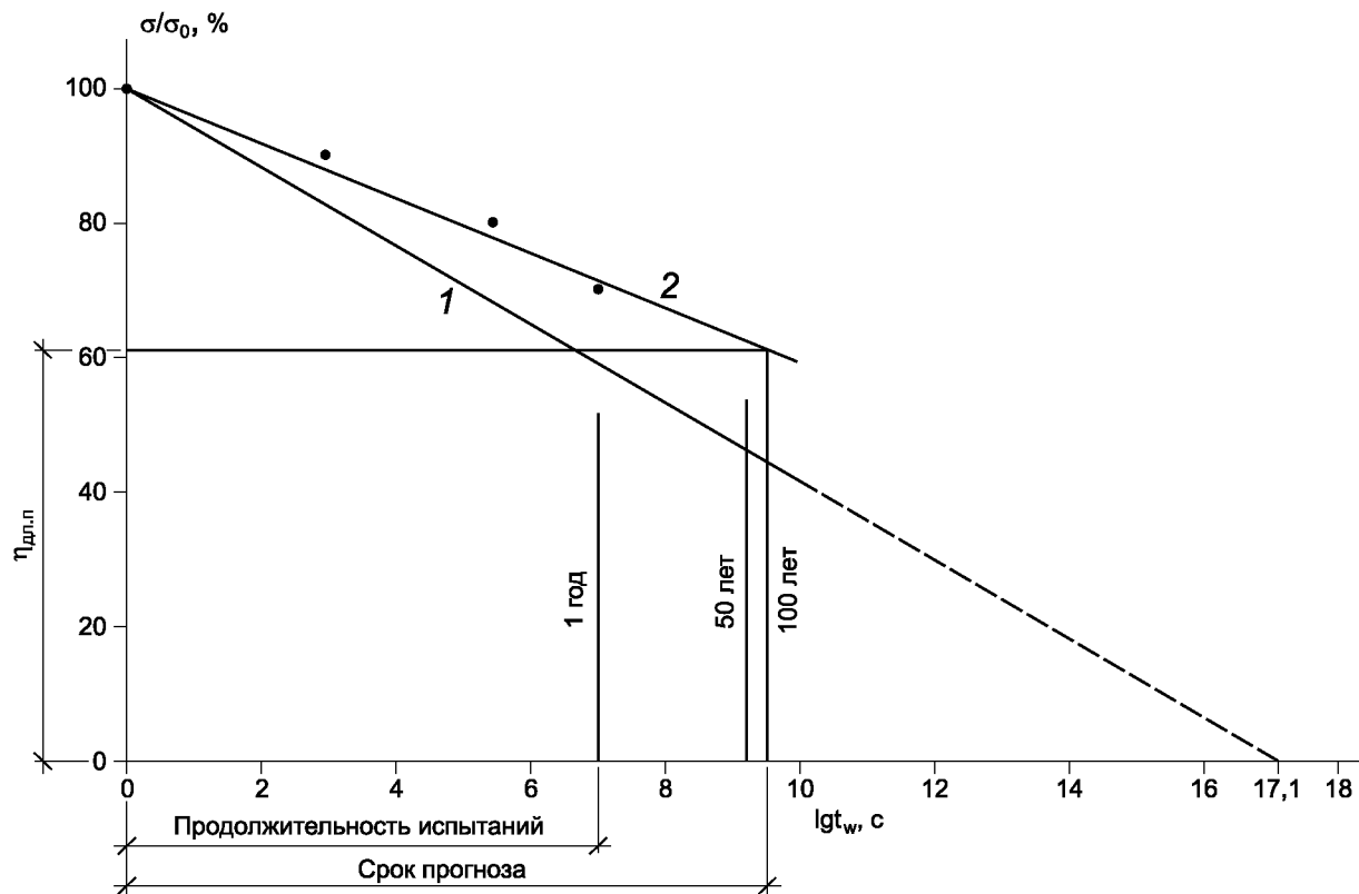
Рисунок 2 — Пример графика временной зависимости прочности от значения приложенной нагрузки
