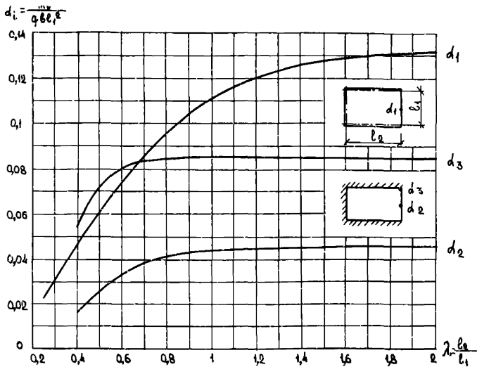
Рис.8. Коэффициенты d_i для прямоугольных плит, опертых по трем сторонам: при свободном опирании ( d_1 ) и защемлении ( d_2, d_3 ); при \lambda > 2 значения d_i принимаются как при \lambda = 2
