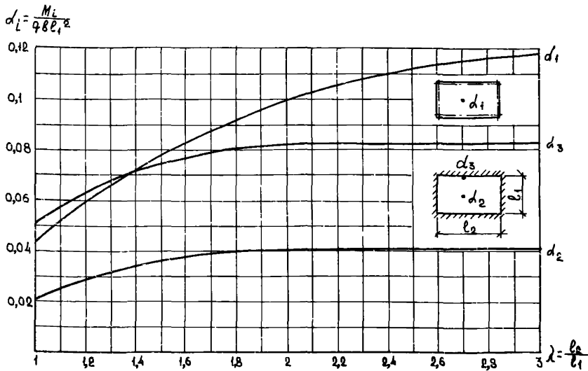
Рис.7. Коэффициенты d_i для прямоугольных плит, опертых по контуру: при свободном опирании ( d_1 ) и защемлении ( d_2, d_3 )
