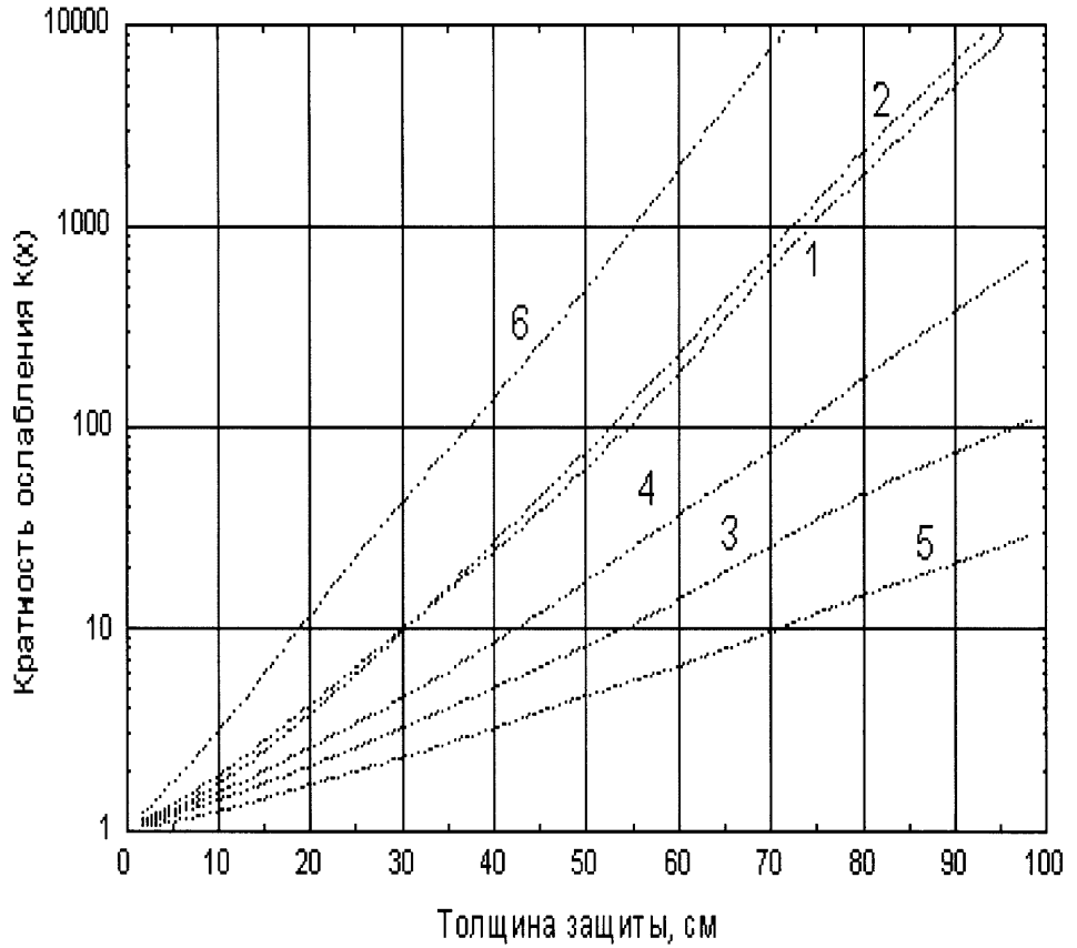
Рисунок В.1 - Зависимость кратности ослабления поглощенной дозы нейтронов от толщины защиты.
