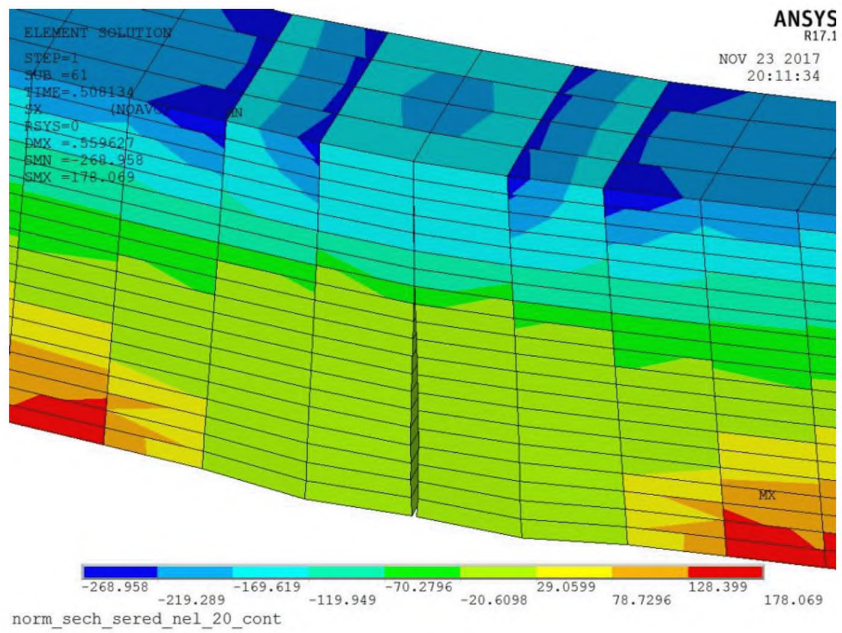
Рисунок П.12 – Фрагмент средней части балки в предельном состоянии. Большие напряжения находятся в упругой части модели
