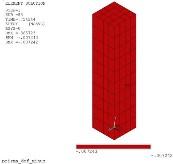
Рисунок П.3 – Относительные вертикальные деформации бетона призмы на последнем шаге нагружения соответствуют предельной величине, заданной в расчетной модели - 2 \times 0,0035
