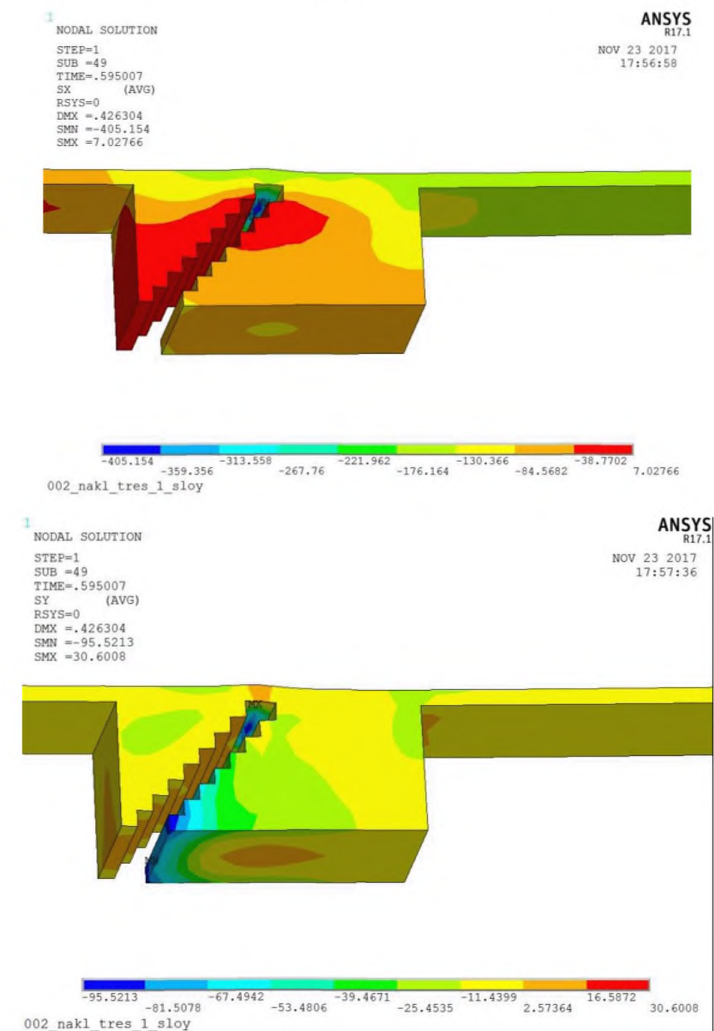
Рисунок П.18 – Горизонтальные и вертикальные нормальные напряжения в нелинейной части балки в окрестности наклонной трещины
