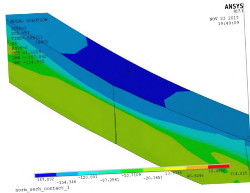
Рисунок П.8 – Фрагмент балки в предельном состоянии. Видна раскрытая трещина. Предельная нагрузка соответствует СП
