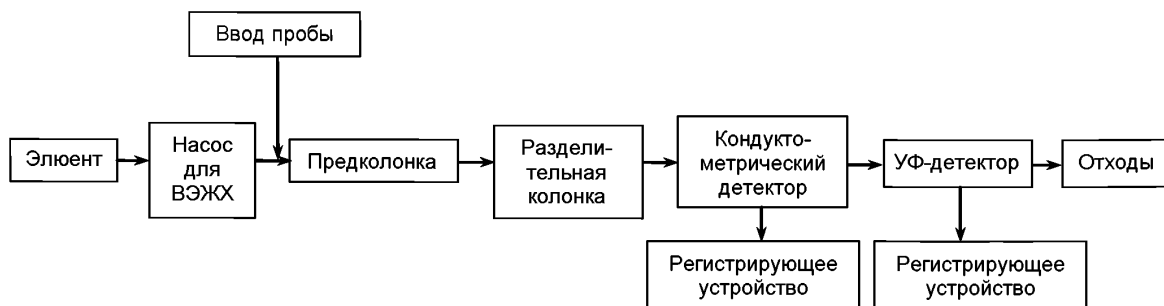
Рисунок 1 — Схема ионной хроматографической системы
