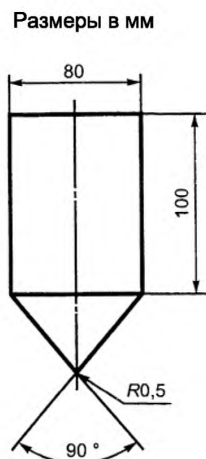
Рисунок 6 – Испытательный конус
