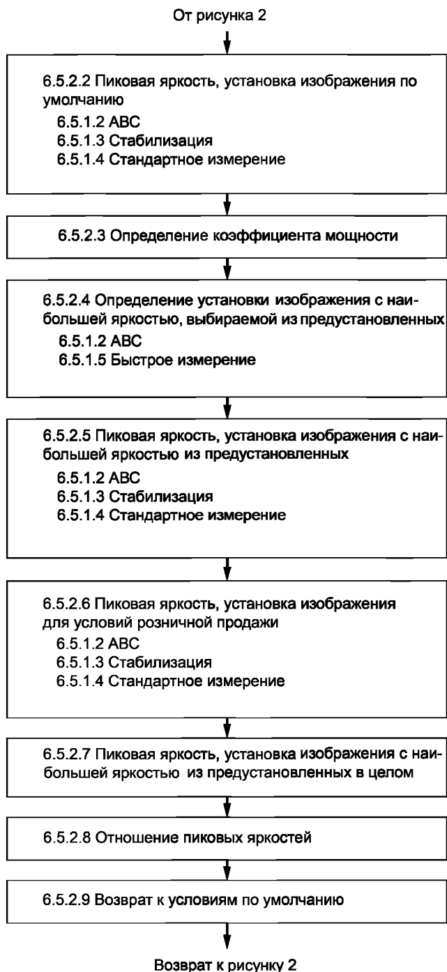
Рисунок 6 — Последовательность действий при определении отношения пиковых яркостей и коэффициента мощности
