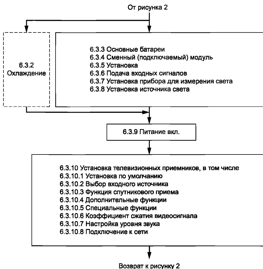
Рисунок 3 — Последовательность первоначальных действий
