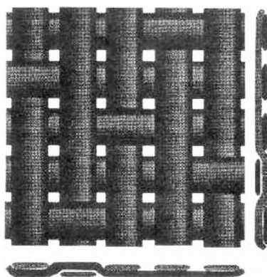
Рисунок 3 — Углеродная ткань сатинового переплетения
