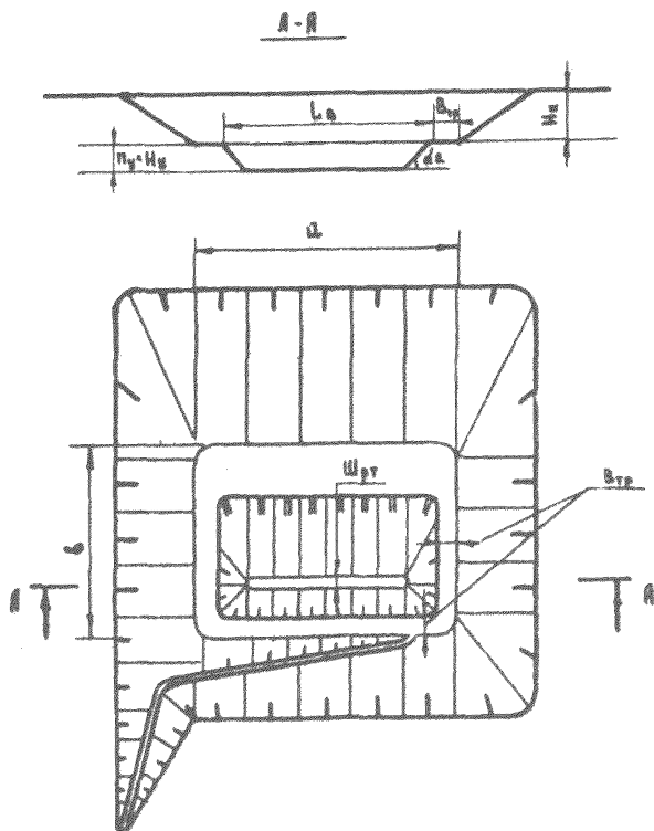
Рис.1. Схема первоначального карьера для расчета его объема и вскрываемой площади по полезному ископаемому.
