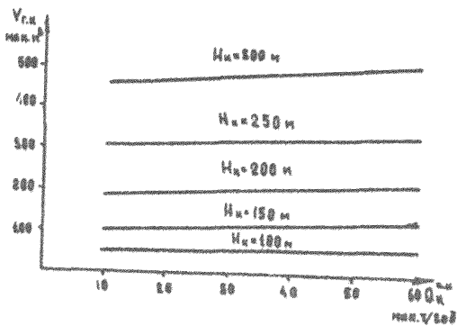
Рис.3. Зависимость объема горно-капитальных работ от производительной мощности карьера.
