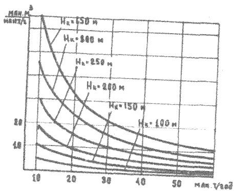
Рис.4. Отношение объемов горно-капитальных работ к производительной мощности карьера.
