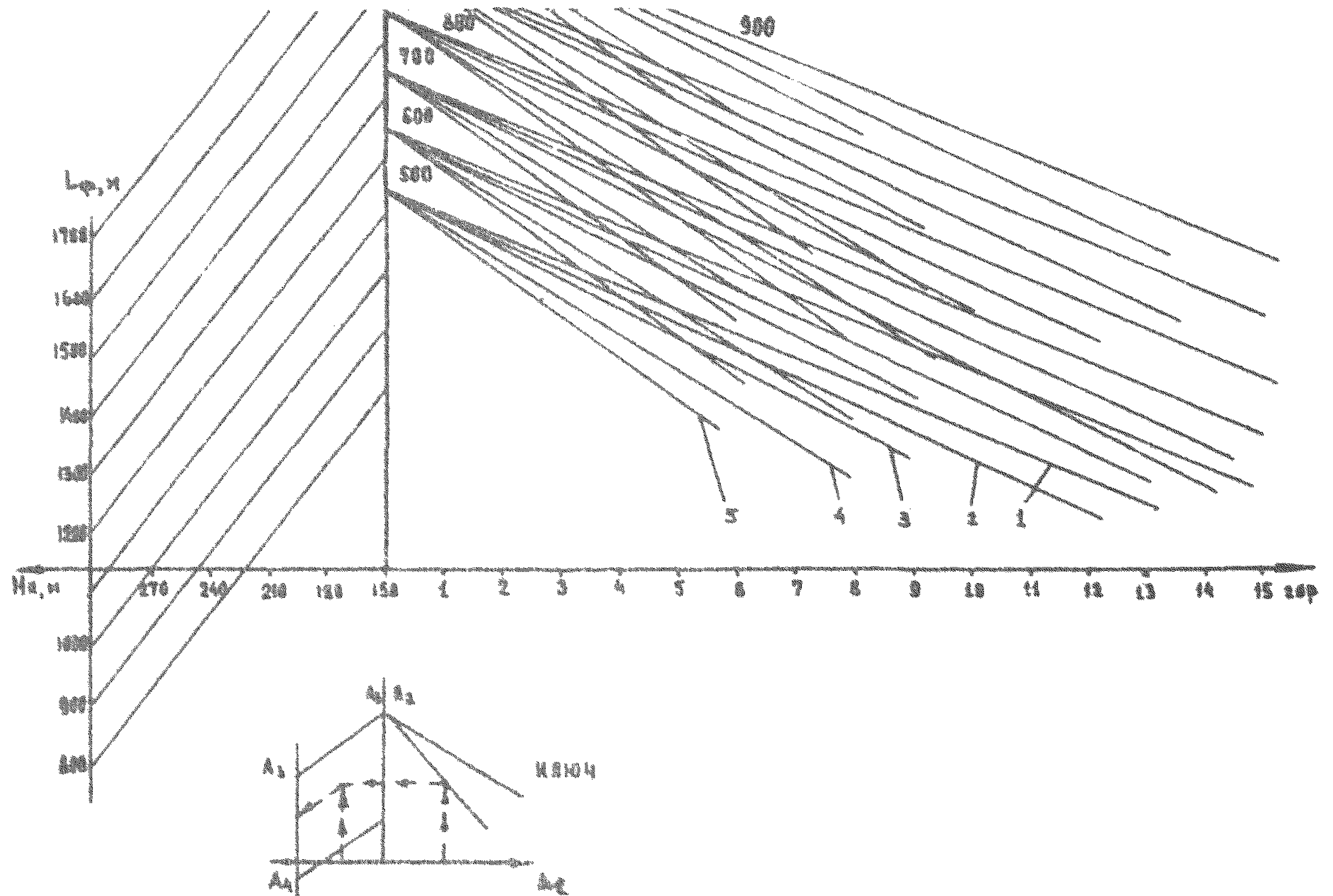
Рис. 10. Номограмма определения протяженности фронта работ на горизонте при различной длине карьера по дну и его глубине
