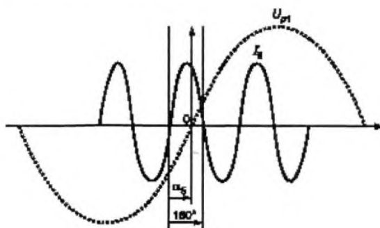
Рисунок 1 – Определение угла фазового сдвига гармонической составляющей тока 5-го порядка I_5 относительно основной составляющей фазового напряжения U_{p1} ( U_{p1}, U_5 > 0 )
