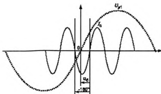
Рисунок 2 – Определение угла фазового сдвига гармонической составляющей тока 5-го порядка I_5 относительно основной составляющей фазового напряжения U_{p1} ( I_5 отстает от U_{p1} , U_5 < 0 )
