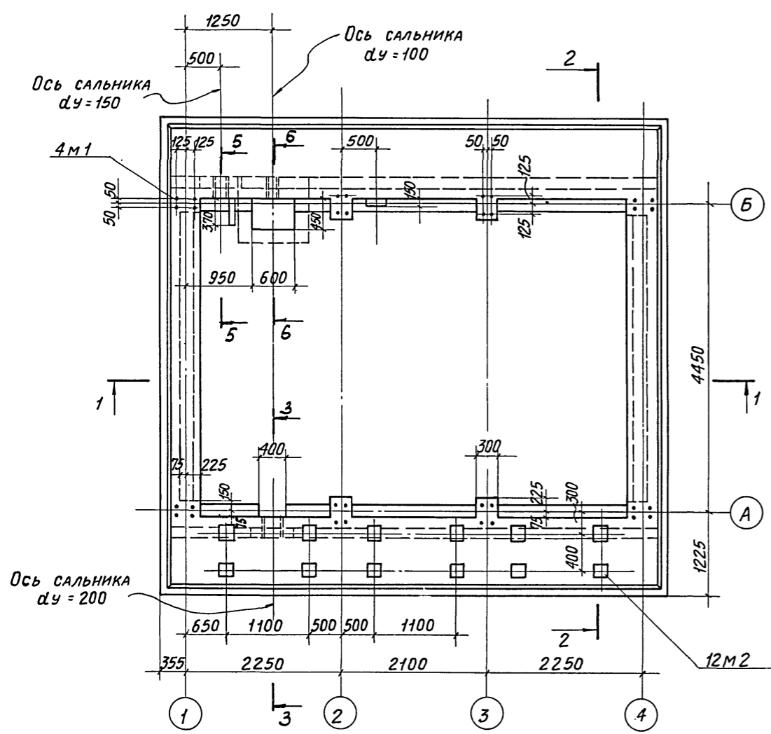
Опалубочный план на отм. 0.000
