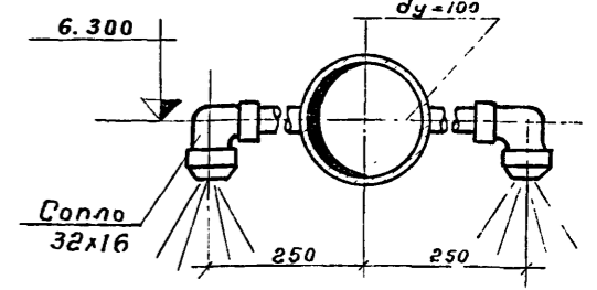
Разрез 4-4 м 1:10
