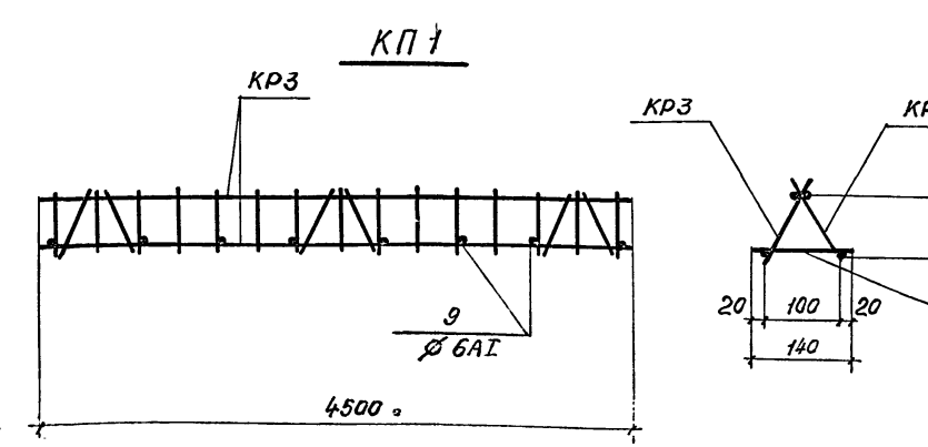
Выборка арматурных изделий на один пространственный каркас
