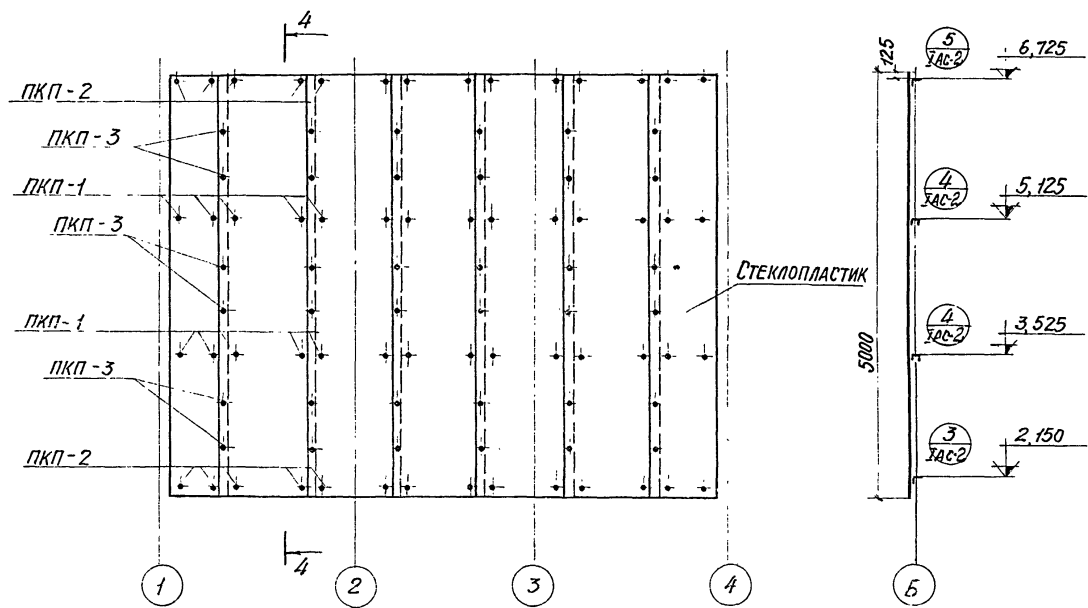
План обшивки из стеклопластика
