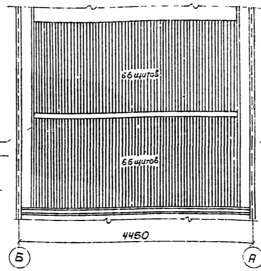
Разрез 2-2
