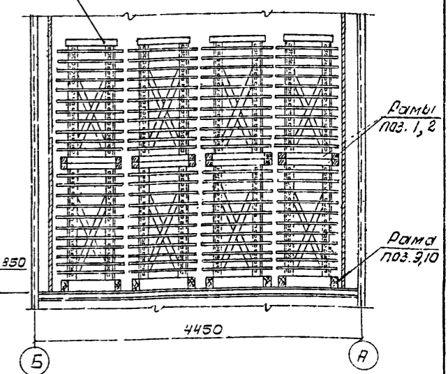
Разрез 4-4
