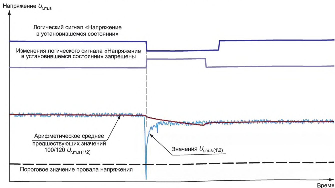
Рисунок 7 — Событие, не относящееся к быстрому изменению напряжения. Пример изменения среднеквадратичного значения напряжения, которое не является событием RVC, так как превышает пороговое значение провала напряжения
