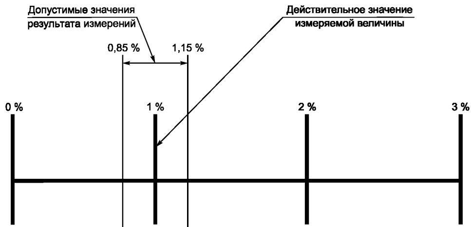
Рисунок 5 — Пример неопределенности измерений несимметрии напряжений
