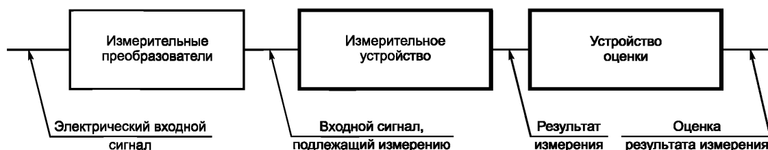
Рисунок 1 — Полная измерительная цепь
