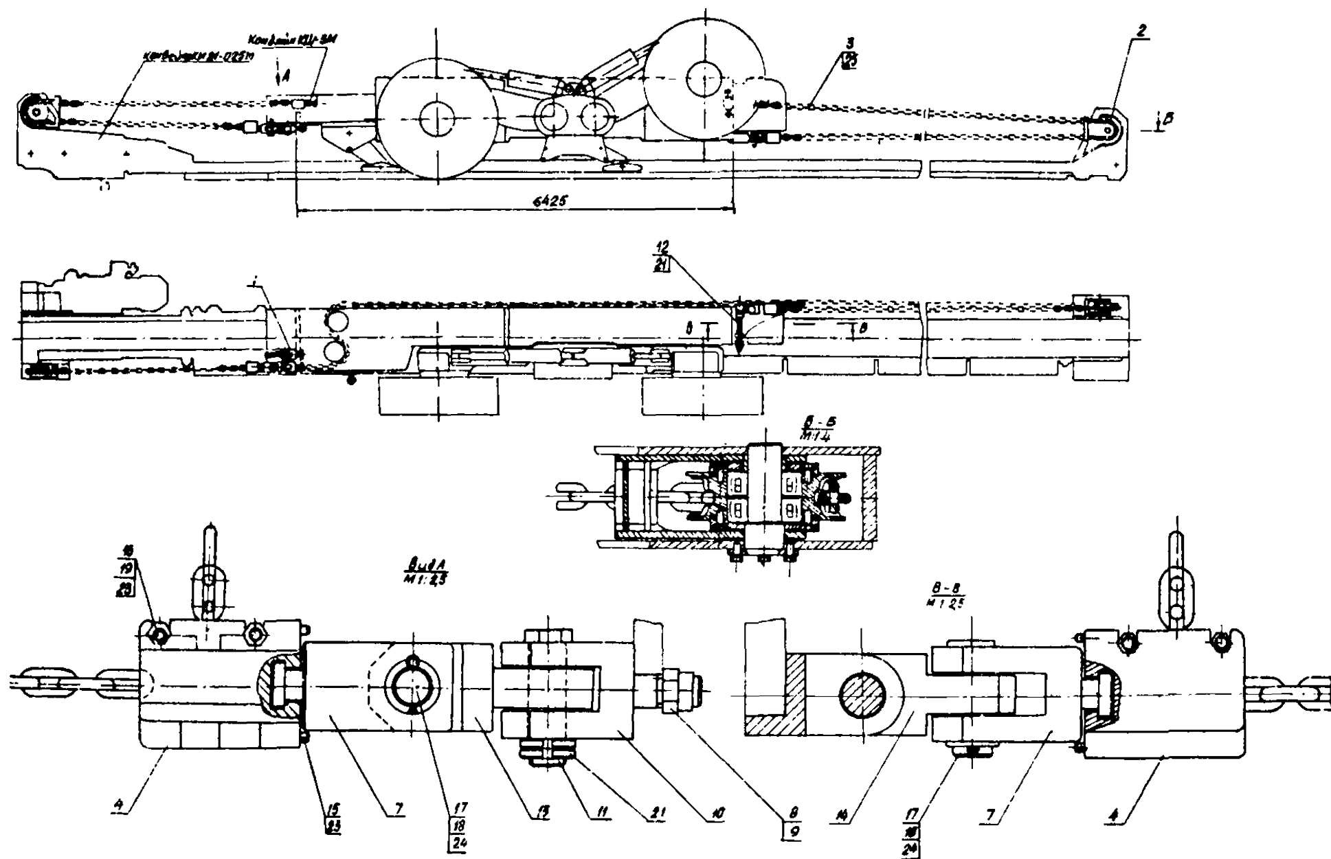
Рис. 3.9. Тяговое устройство
