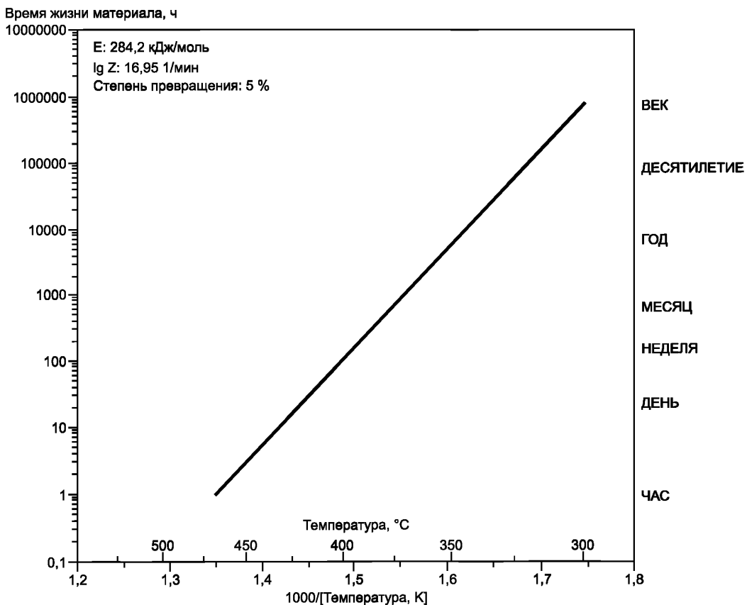
Рисунок 1 — Кривая термической устойчивости
