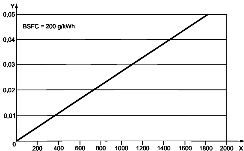
Рисунок 1 — Соотношение между содержанием серы в топливе и выбросами сульфатов в двигателях без системы каталитической очистки отработавших газов
