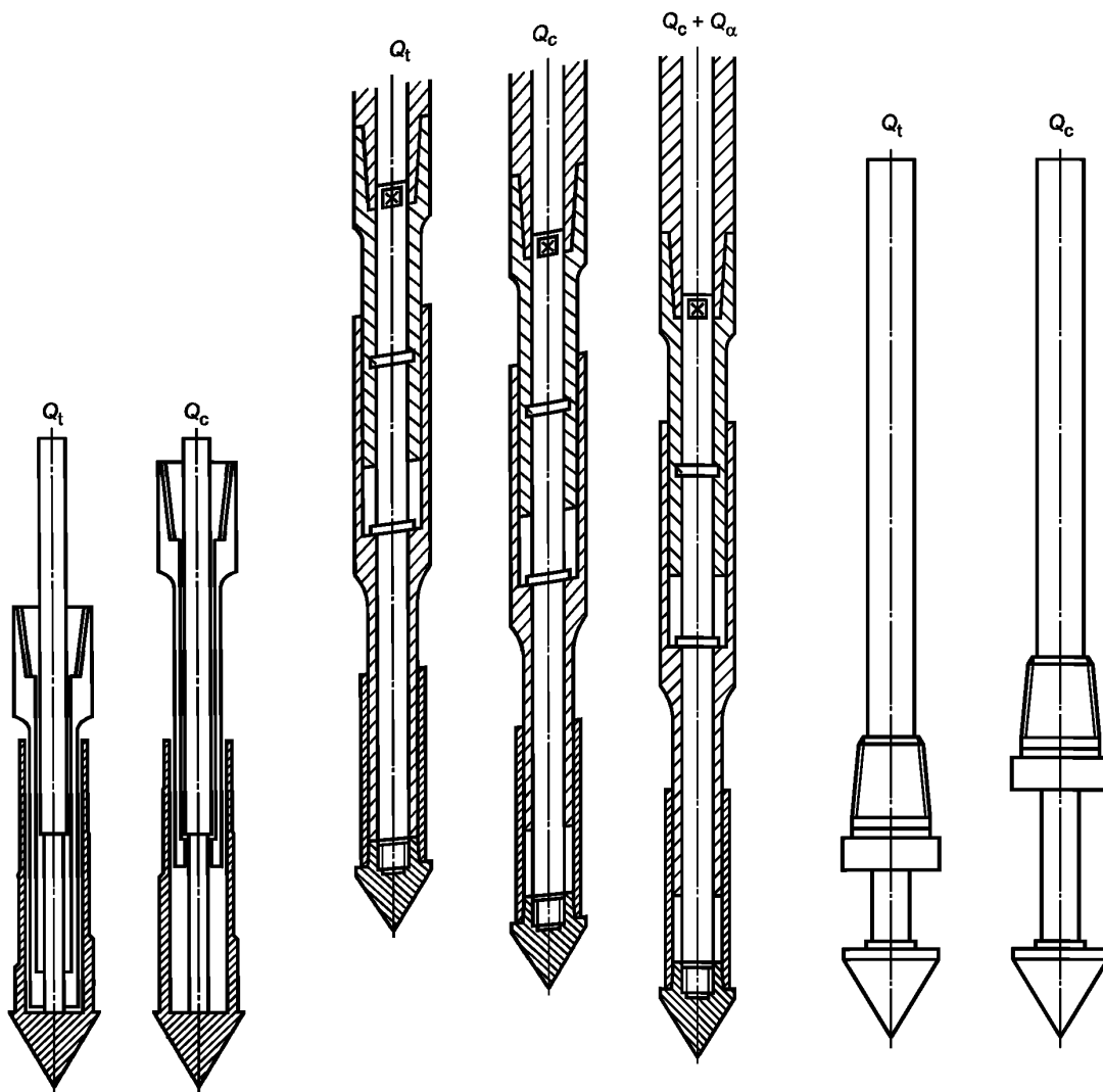
Рисунок 4 — Наконечник M4 (простой конус)
