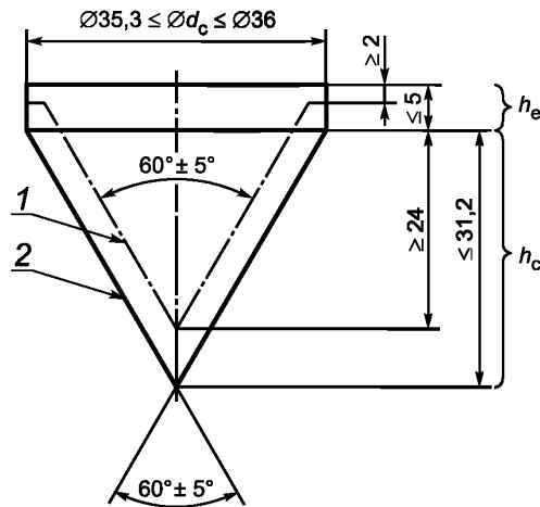
Рисунок 5 — Требования к допускам при применении наконечника
