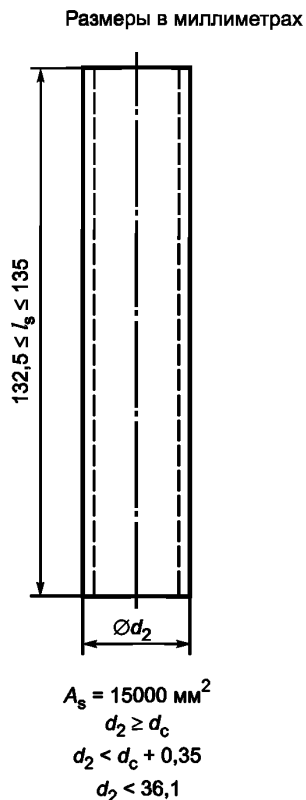
Рисунок 6 — Требования к допускам для муфты трения
