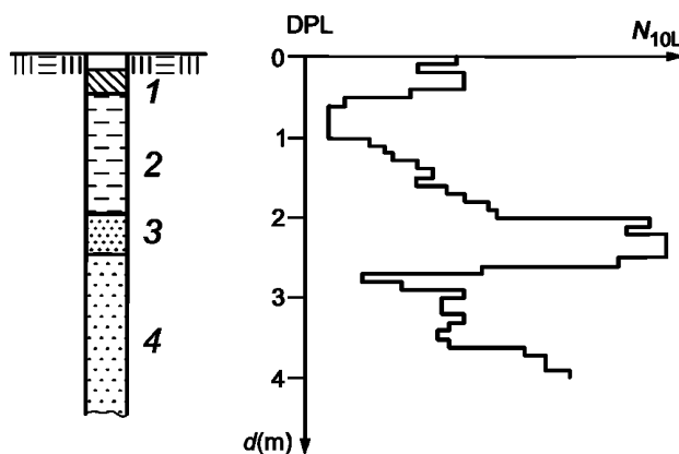
1 — суглинок; 2 — глина; 3 — среднезернистый песок (цементированный); 4 — среднезернистый песок; d — глубина
