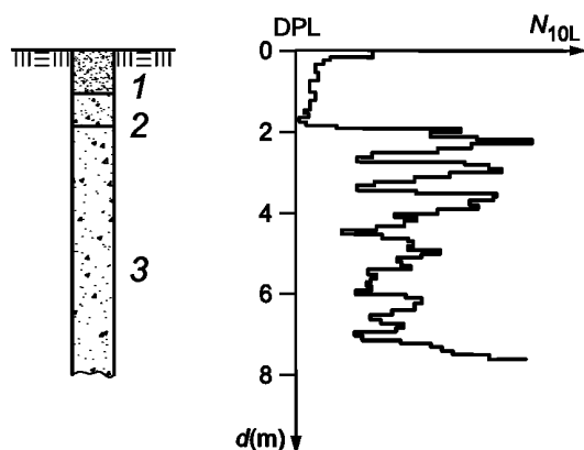
1 — супесь, песчаная; 2 — супесь; 3 — гравий; d — глубина
