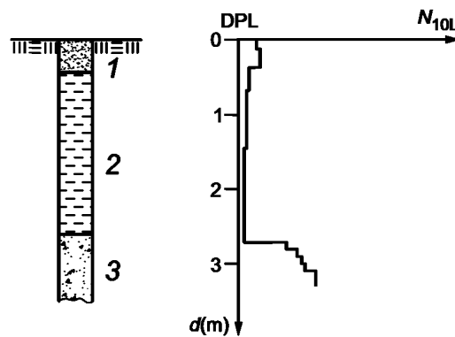
1 — пылевая глина; 2 — торф (разложившийся); 3 — глина (песчаная, высокая степень пылеватости); d — глубина
