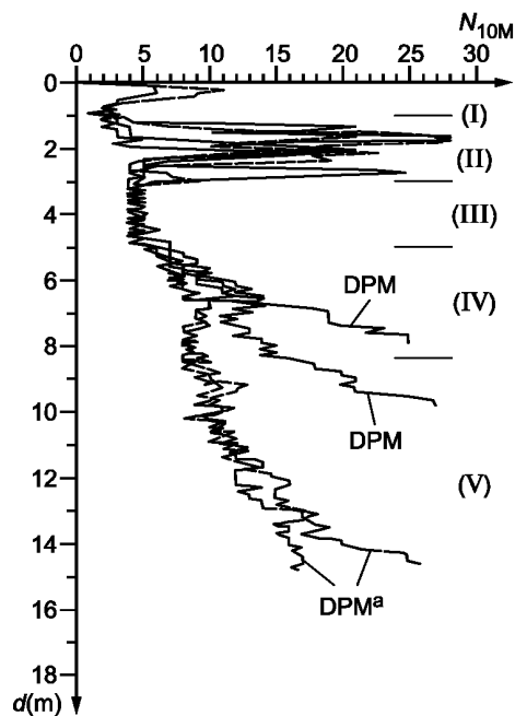
DPM — динамическое зондирование без бурового раствора; DPM a — динамическое зондирование с буровым раствором; I — почва; II — гравий; III — переработанная выветренная глина; IV — выветренная глина; V — невыветренная глина; d — глубина
