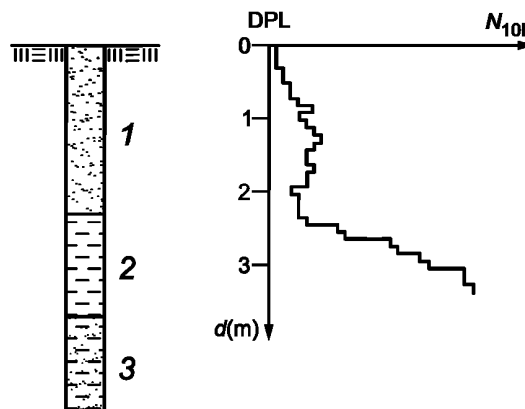
1 — гравий и песок; 2 — торф (волокнистый); 3 — мелкий песок и супесь (слабоглинистые); d — глубина
