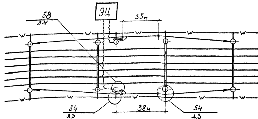
Электрическая схема подключения аппаратуры
