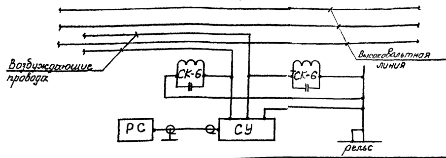
Электрическая схема подключения аппаратуры
