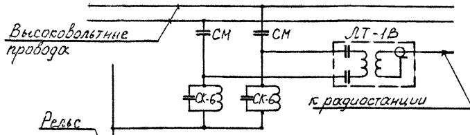
Высоковольтные провода Рельс Проводов ДПР, расположенных с разных сторон путей
