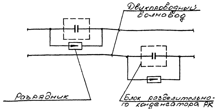
Электрическая схема подключения аппаратуры двухпроводного волновода
