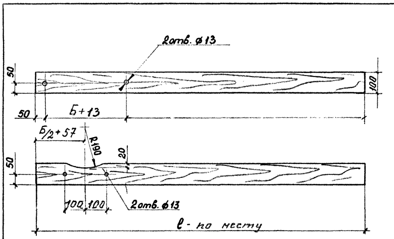
Б-база железобетонной опоры (Б-см. черт.4484-46).
