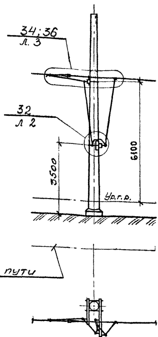
Однопроводный волновод
