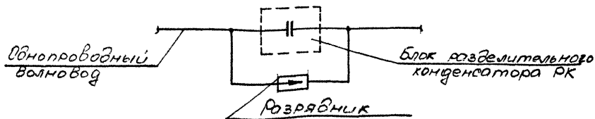
Электрическая схема подключения аппаратуры однопроводного волновода
