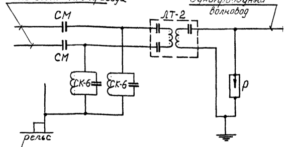
Электрическая схема подключения аппаратуры высоковольтные провода
