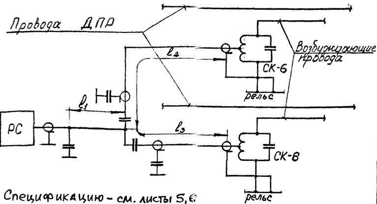
Электрическая схема подключения аппаратуры
