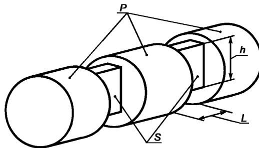
Рисунок 2 — Эскиз образцов с приклеенными накладками
