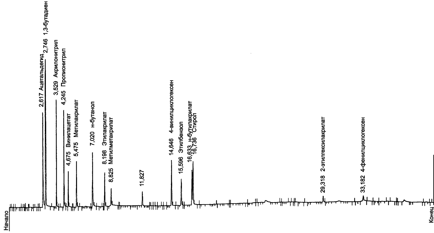
Рисунок 1 — Типовая хроматограмма
