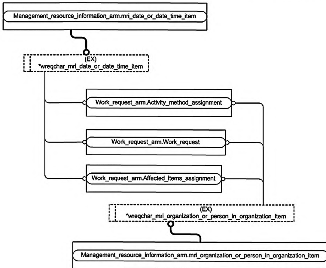
Рисунок С.4 — Представление ПЭМ на уровне объектов в формате EXPRESS-G. Диаграмма 3 из 4
