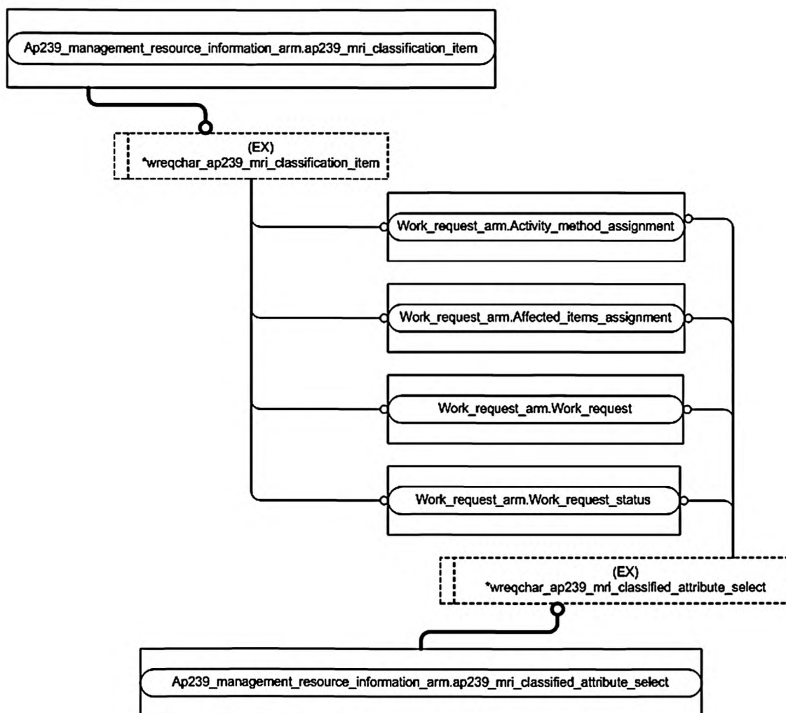
Рисунок С.2 — Представление ПЭМ на уровне объектов в формате EXPRESS-G. Диаграмма 1 из 4
