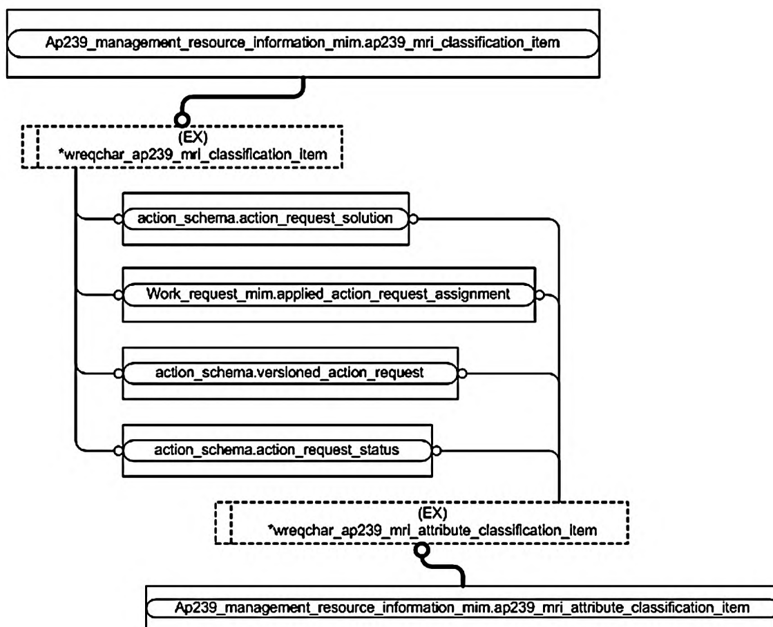
Рисунок D.2 — Представление ИММ на уровне объектов в формате EXPRESS-G. Диаграмма 1 из 5
