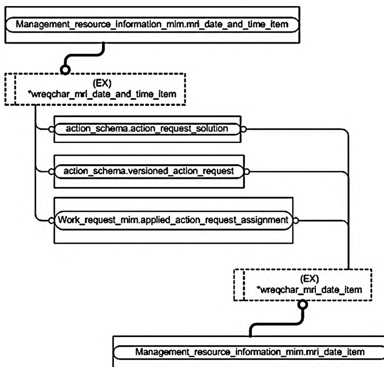
Рисунок D.4 — Представление ИММ на уровне объектов в формате EXPRESS-G. Диаграмма 3 из 5
