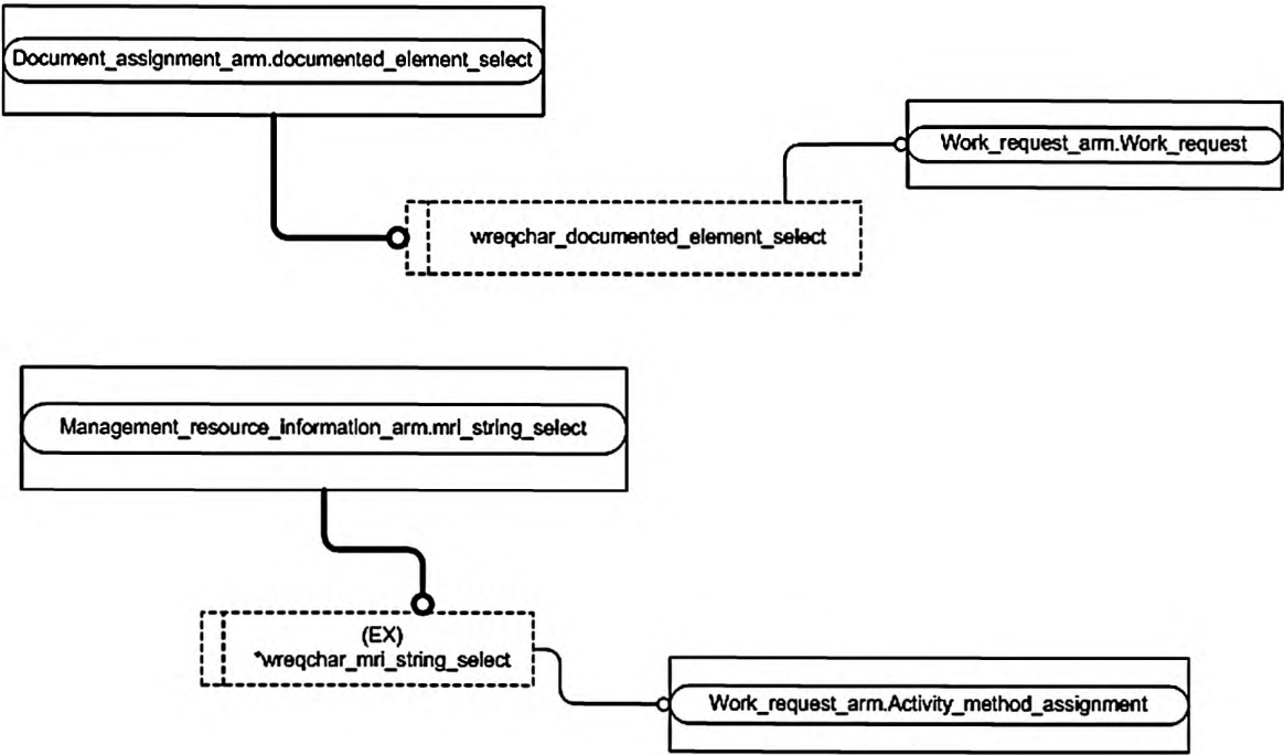
Рисунок С.5 — Представление ПЭМ на уровне объектов в формате EXPRESS-G. Диаграмма 4 из 4
