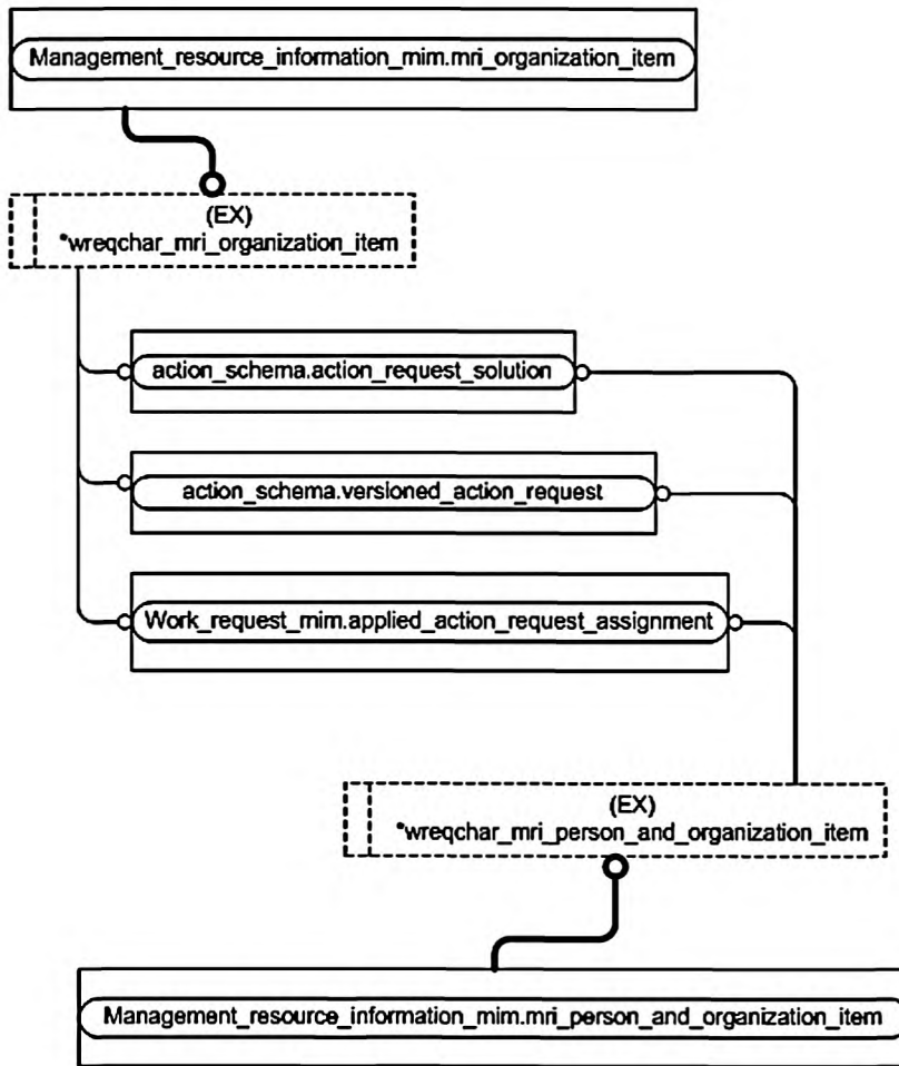
Рисунок D.5 — Представление IMM на уровне объектов в формате EXPRESS-G. Диаграмма 4 из 5
