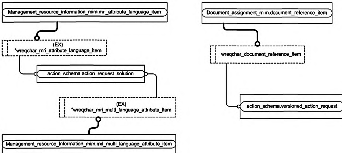
Рисунок D.6 — Представление IMM на уровне объектов в формате EXPRESS-G. Диаграмма 5 из 5
