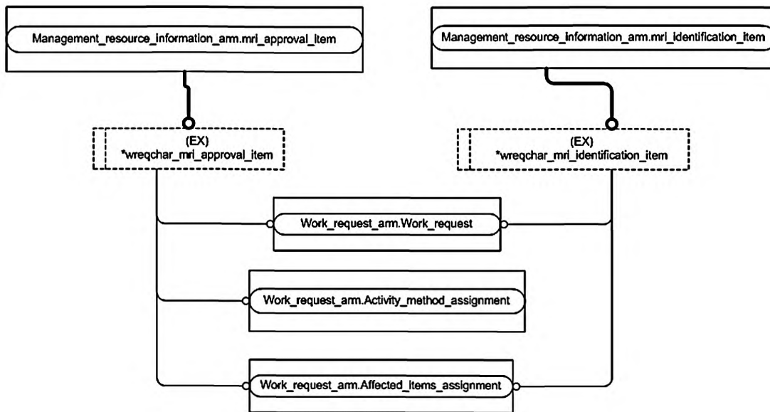
Рисунок С.3 — Представление ПЭМ на уровне объектов в формате EXPRESS-G. Диаграмма 2 из 4
