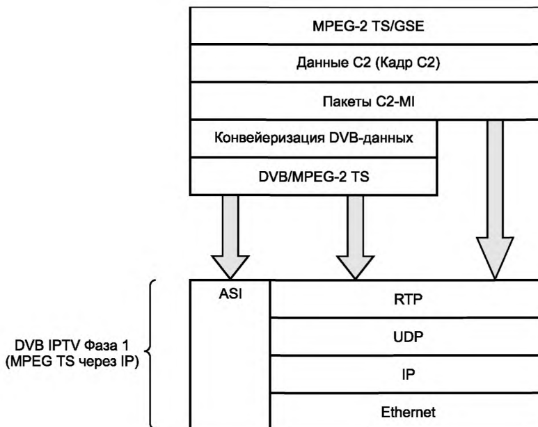
Рисунок 2 — Стек протоколов C2-MI
