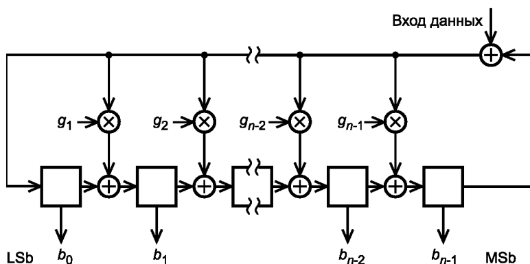
Рисунок А.1 — Схема генерации CRC
