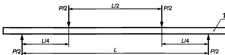
Рисунок 3 — Четырехточечный изгиб
