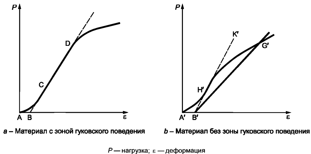
Рисунок А2.1 — Графики зависимости «нагрузка—деформация»
