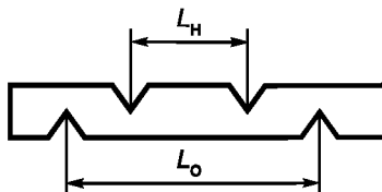
Рисунок А1.3 — Шаблон для установки опор
