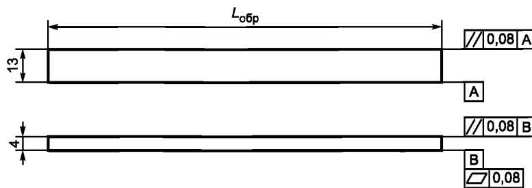
Рисунок 1 — Образец для испытаний
