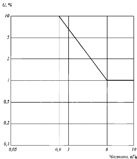
Рис. 5.1.43.3.2 Кривая испытательного напряжения при проверке оборудования на устойчивость к низкочастотным кондуктивным помехам
