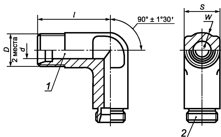
1, 2 — наконечник
