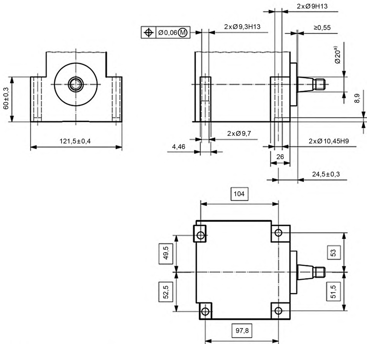
Рисунок 8 — Трехсекционный топливный насос высокого давления с установкой на основание, исполнение 8
